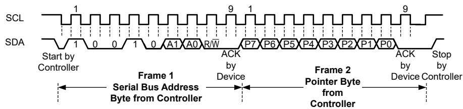
图 7-2. 针对写入指针字节的两线制时序图
