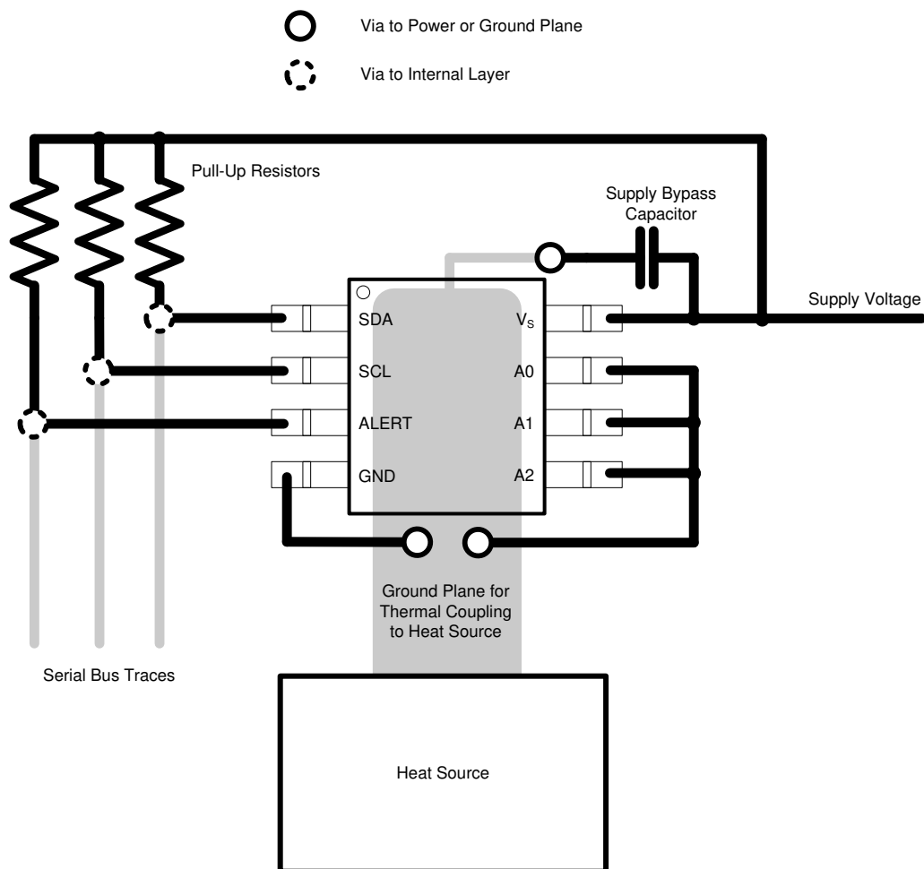
图 9-3. 布局示例
