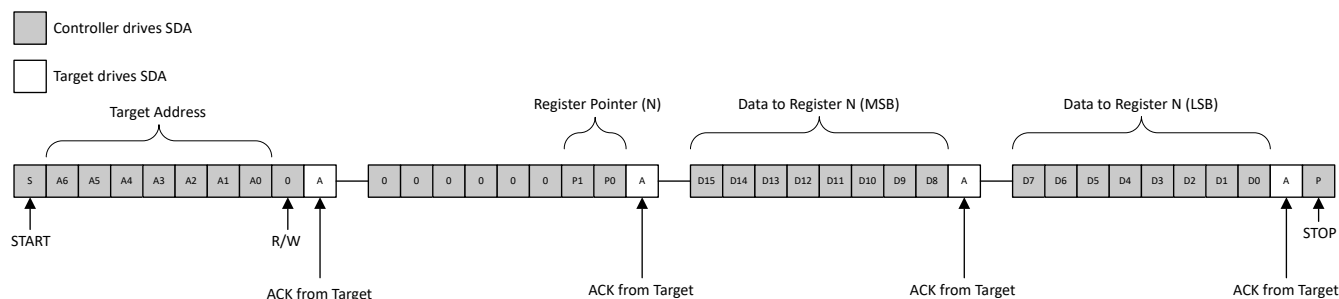
图 7-2. 两线制时序图
