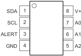
图 5-1. DGK 和 D 封装 8 引脚 VSSOP 和 SOIC 顶视图
