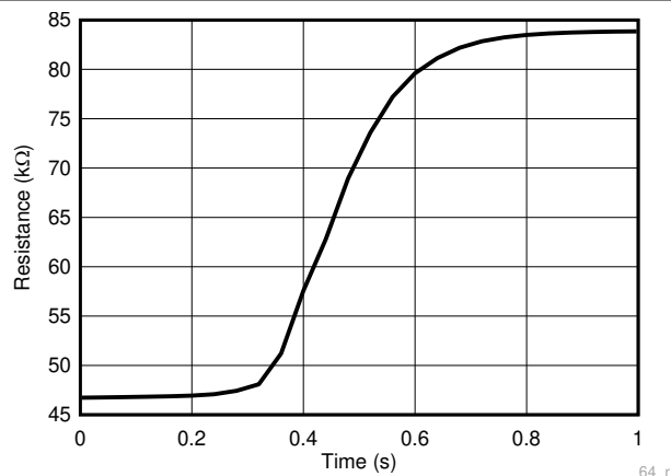
图 7-8. DEC 热响应时间
