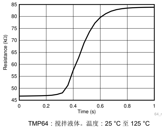
图 7-9. DYA 热响应时间
