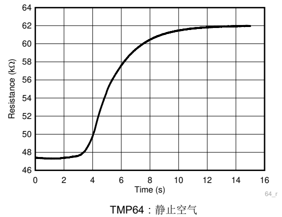
图 7-10. 热响应时间
