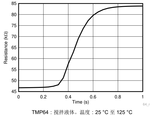
图 7-8. DEC 热响应时间
