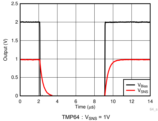
图 7-7. 阶跃响应
