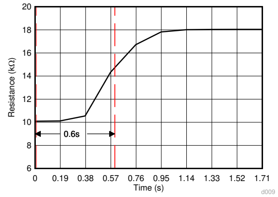
图 6-8. 热响应时间 ( DEC 封装 )
