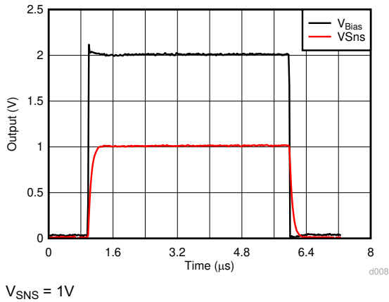
图 6-7. 阶跃响应
