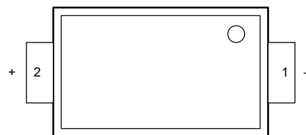
图 5-2. DYA 封装 2 引脚 SOT-5X3 顶视图
