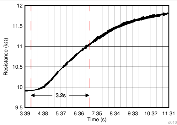
图 6-7. 阶跃响应
