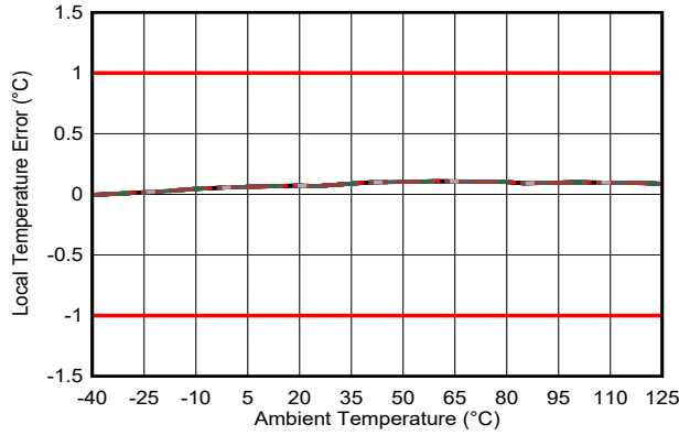
图 7-2. 本地温度误差与温度之间的关系
