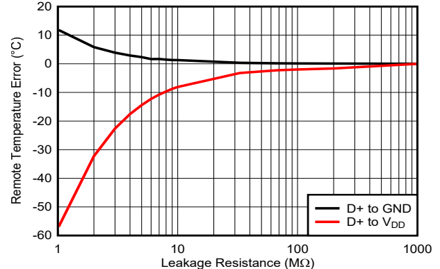
图 7-5. 远程温度误差与二极管并联泄漏电阻之间的关系
