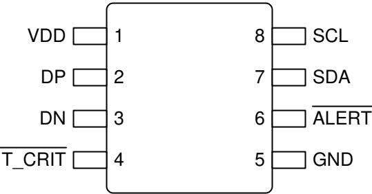
图 6-1. DGK 封装 8 引脚 VSSOP ( 顶视图 )
