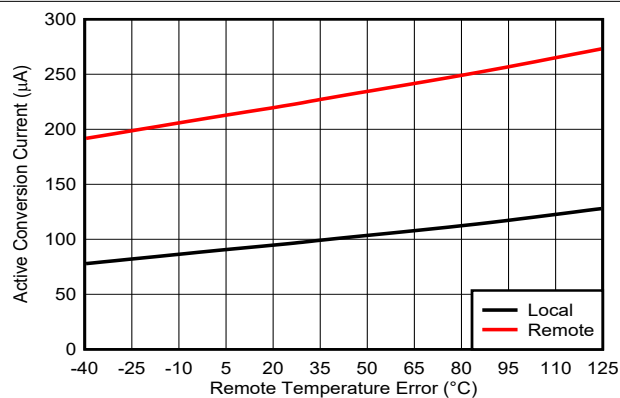
图 7-8. 有效电流与温度间的关系
