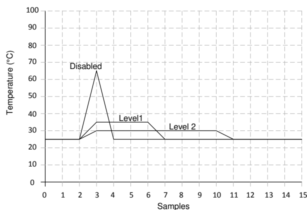
图 8-3. 滤波器对脉冲输入的响应
