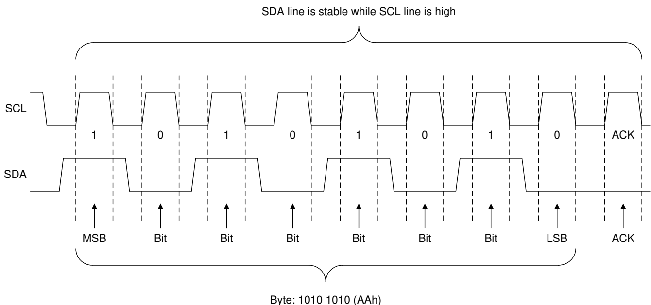
图 8-11. 位传输
