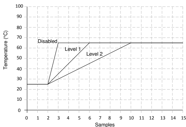
图 8-4. 滤波器对阶跃输入的响应
