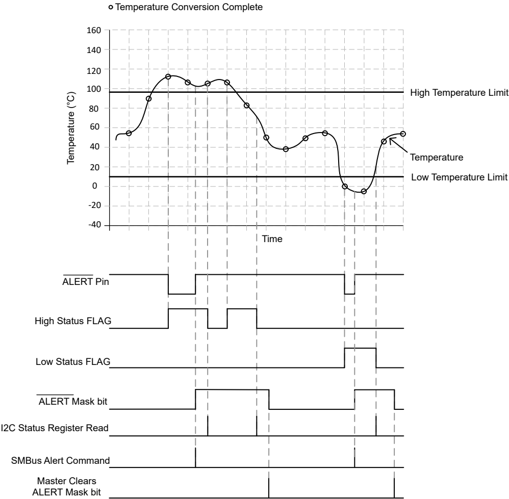
图 8-15. 警报 SMBus 模式时序图
