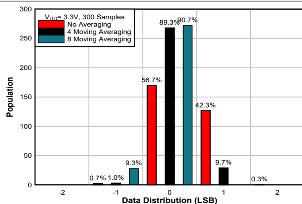
图 7-10. 远程温度噪声数据分布 (300 个样本)
