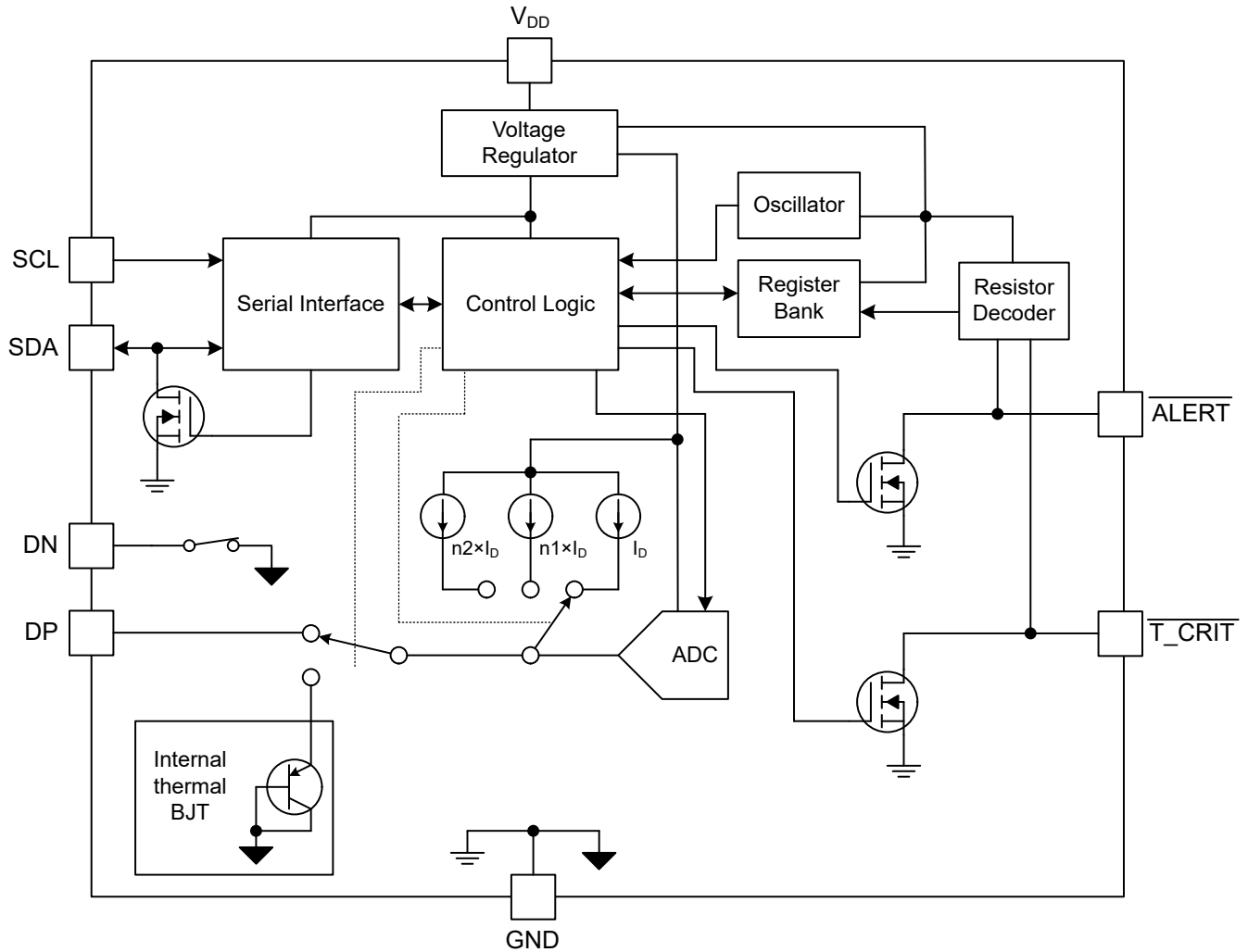
图 8-1. 功能方框图
