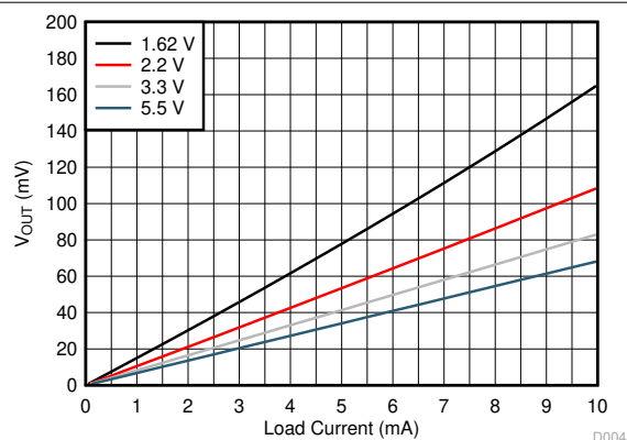
图 6-6. 输出电压与负载电流之间的关系
