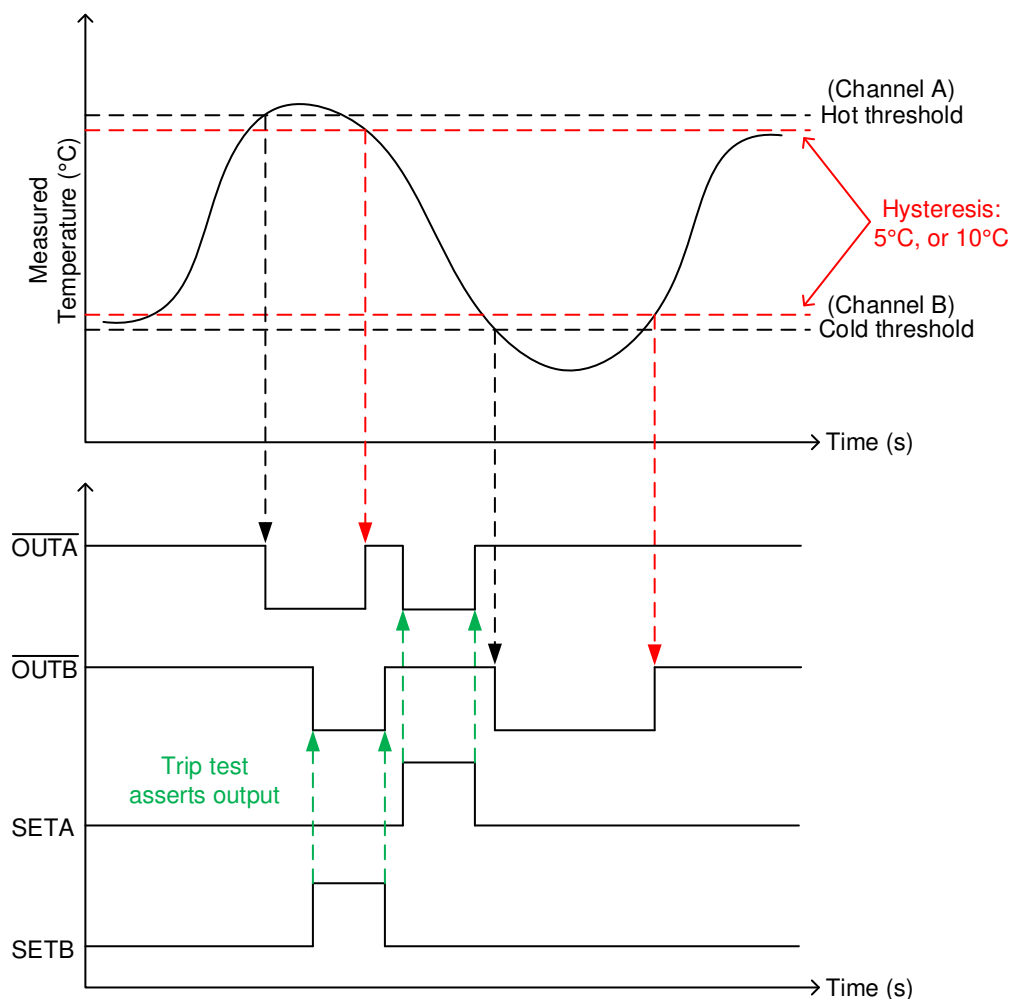
图 7-2. TMP390-Q1 跳闸测试操作
