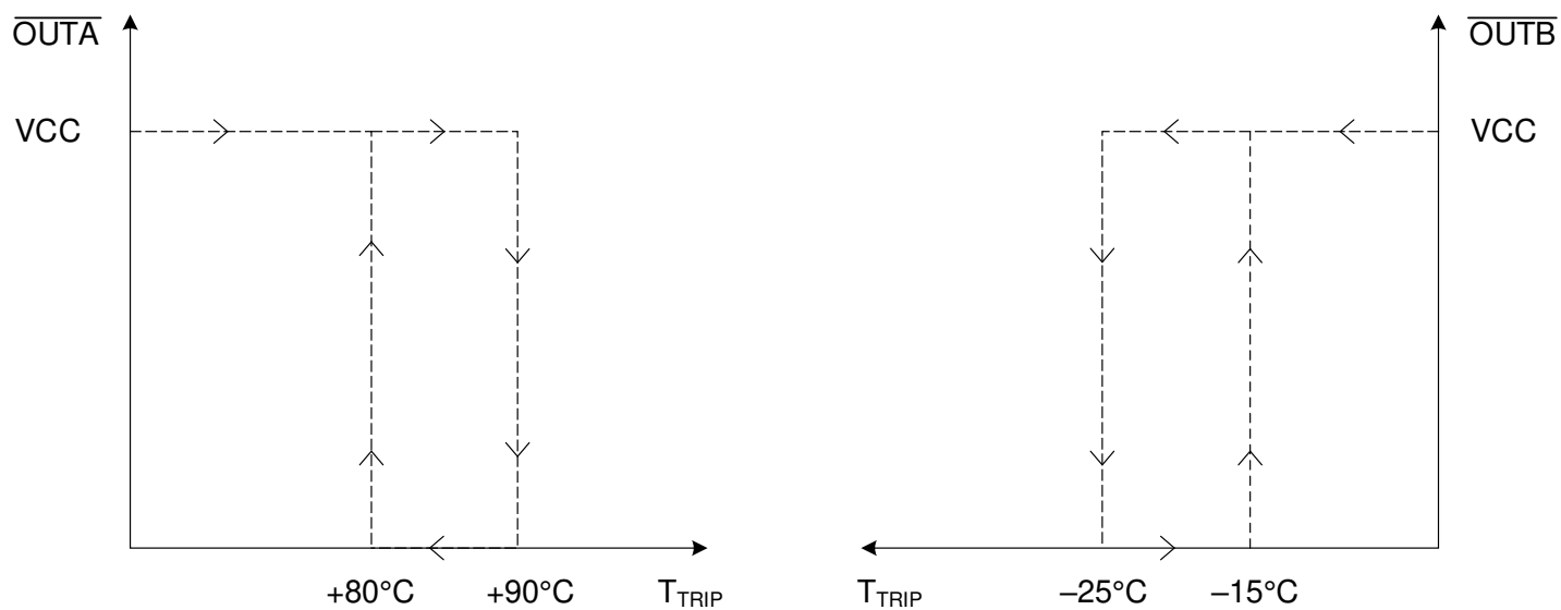
图 8-4. 具有迟滞功能的 TMP390 输出响应
