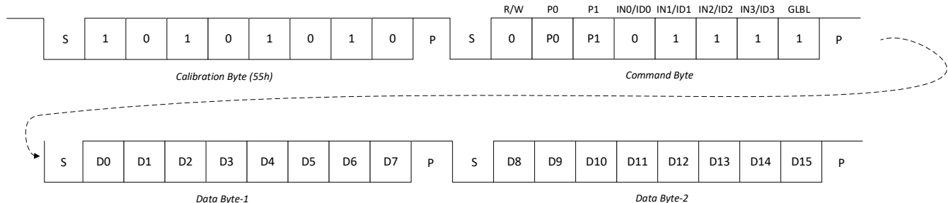
图 7-12. 全局写入命令流程
