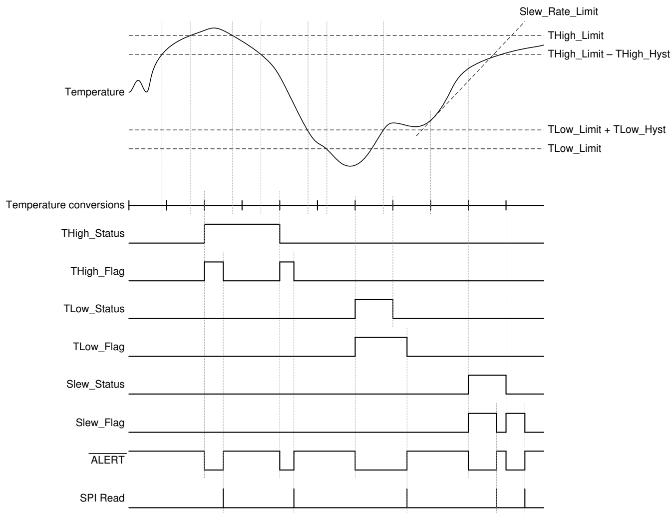
图 8-7. 中断模式图
