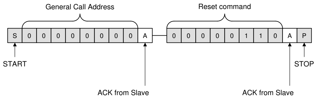
图 7-12. 通用广播复位命令时序图
