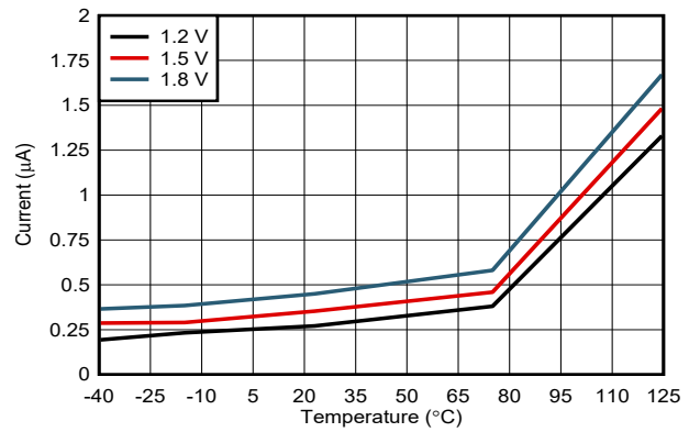
图 7-4. 待机电流与温度间的关系
