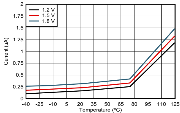
图 7-3. 有效电流与温度间的关系
