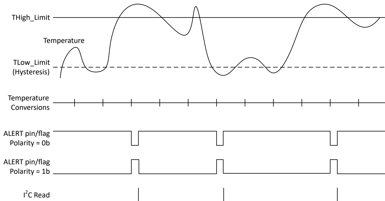
图 7-2. 警报模式
