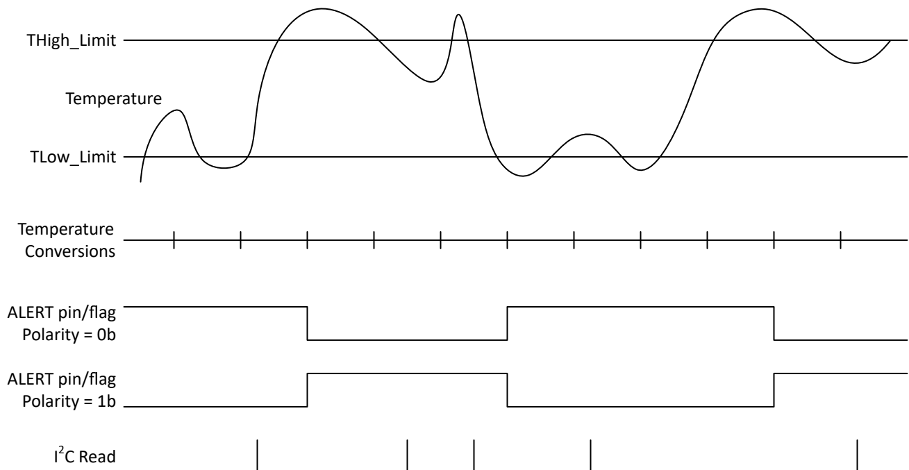
图 7-1. 比较器模式
