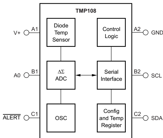
方框图
