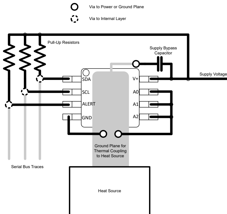
图 12-2. Layout Example (DKG Package)
