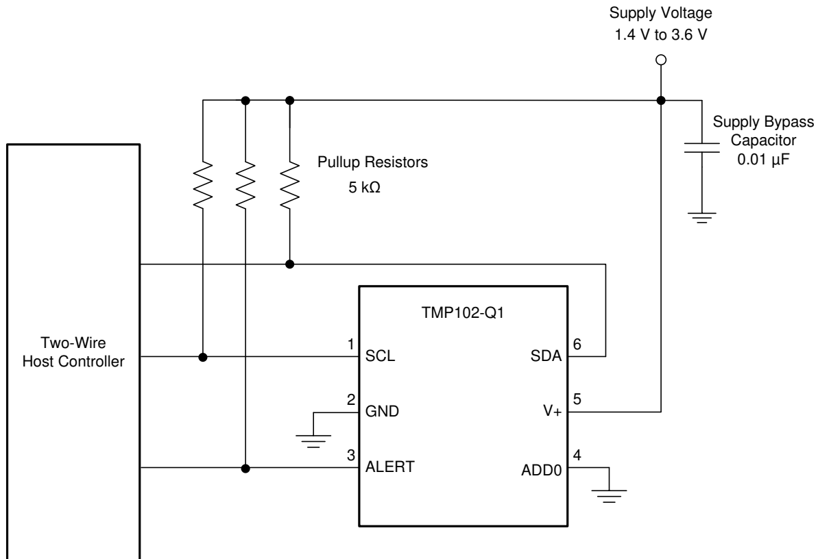
图 8-1. 典型连接
