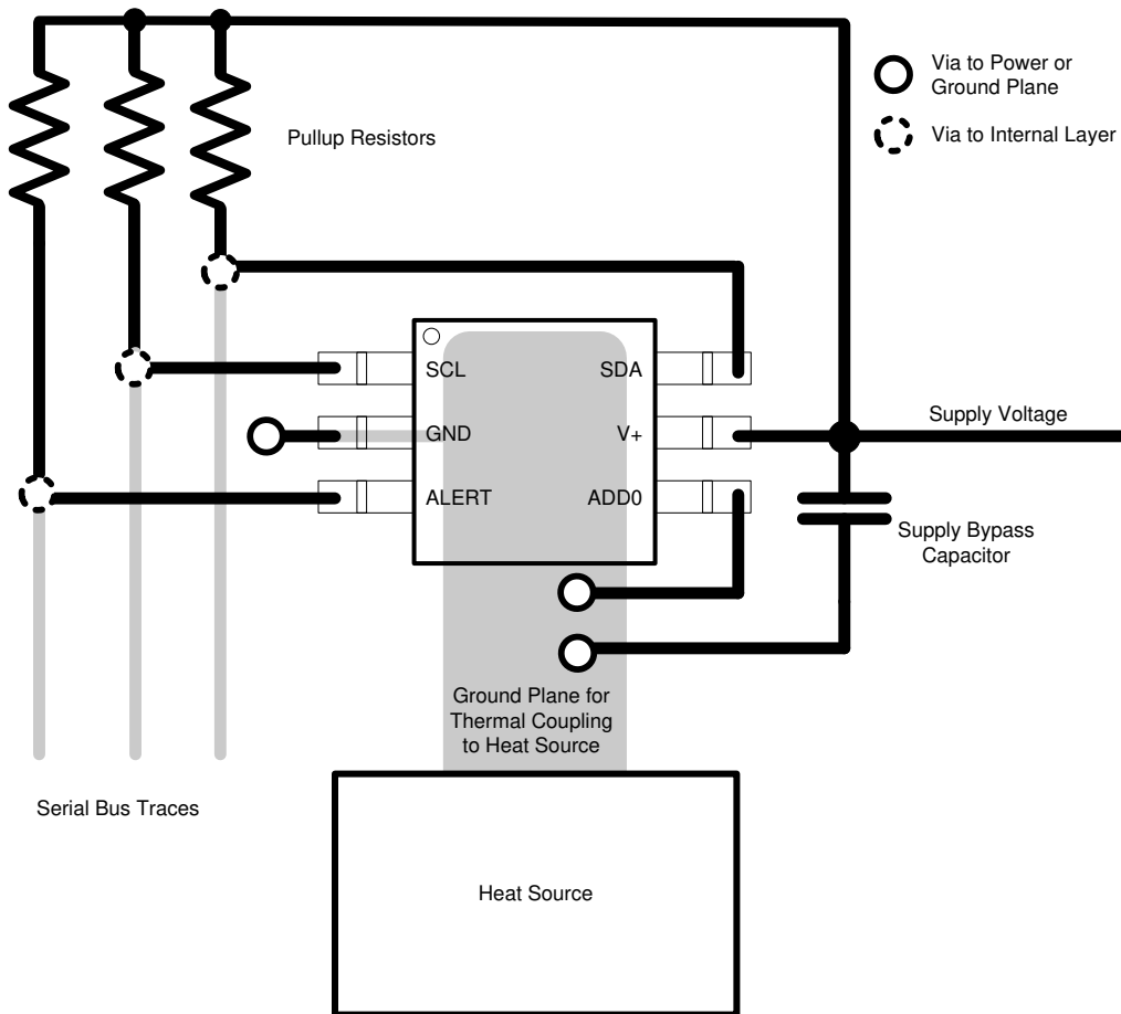
图 10-1. TMP102-Q1 布局示例
