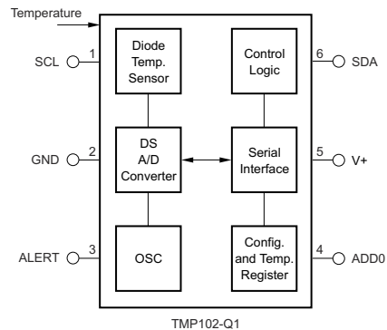
方框图
