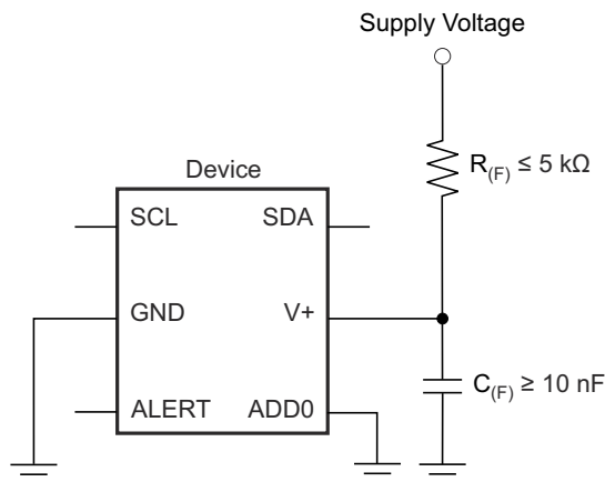
图 8-2. 降噪技术
