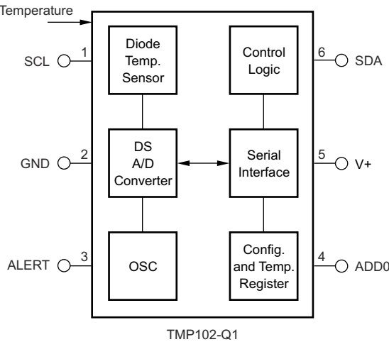
图 7-1. 内部框图
