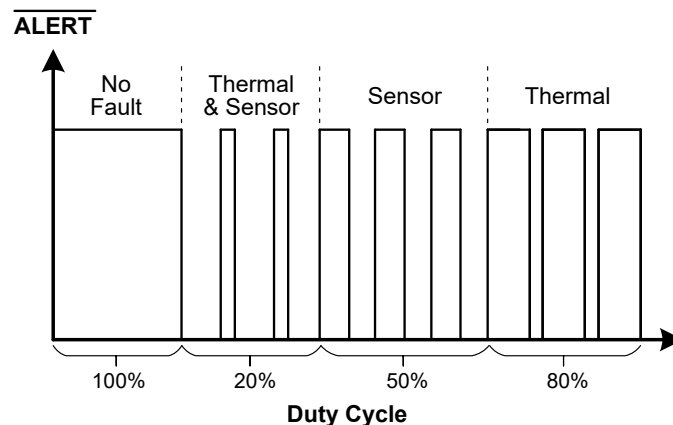
图 9-6. 传感器诊断波形
