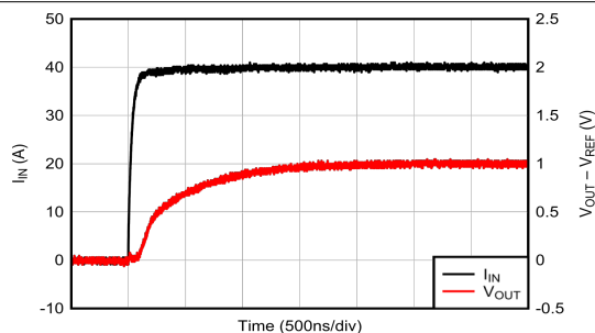
图 7-7. 电压输出阶跃响应 (上升)
