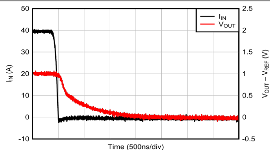
图 7-8. 电压输出阶跃响应 (下降)
