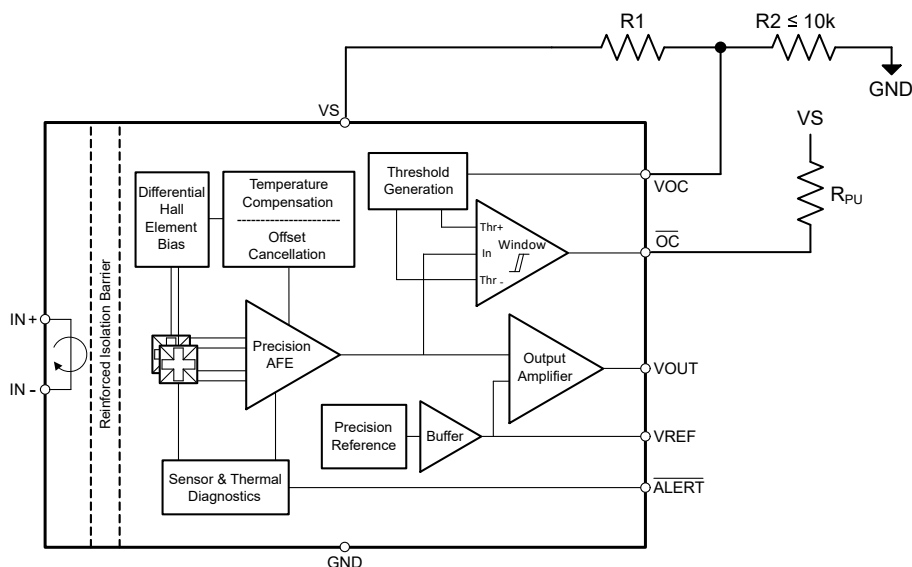
图 9-3. 使用电源电压的用户可配置过流阈值
