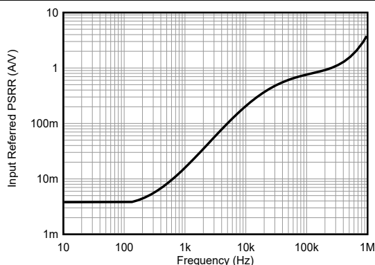
图 7-5. PSRR 与频率间的关系
