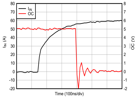
图 7-9. 过流输出响应
