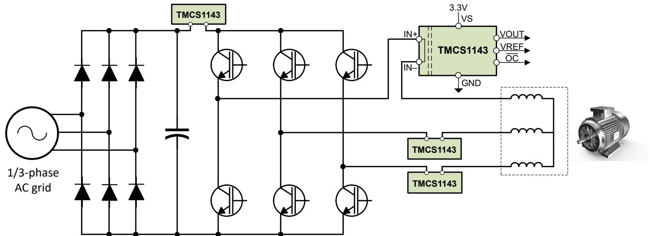
图 10-2. 内嵌式电机相电流检测
