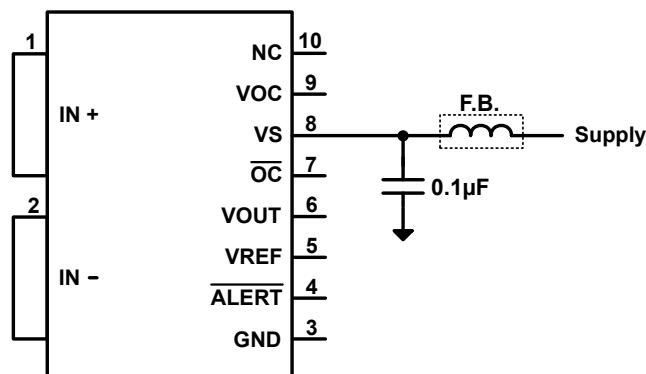
图 10-4. 电源噪声滤波
