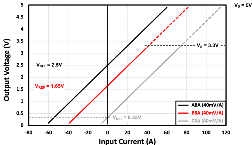
图 9-2. TMCS1143x8A 的输出电压和输入电流间关系。
