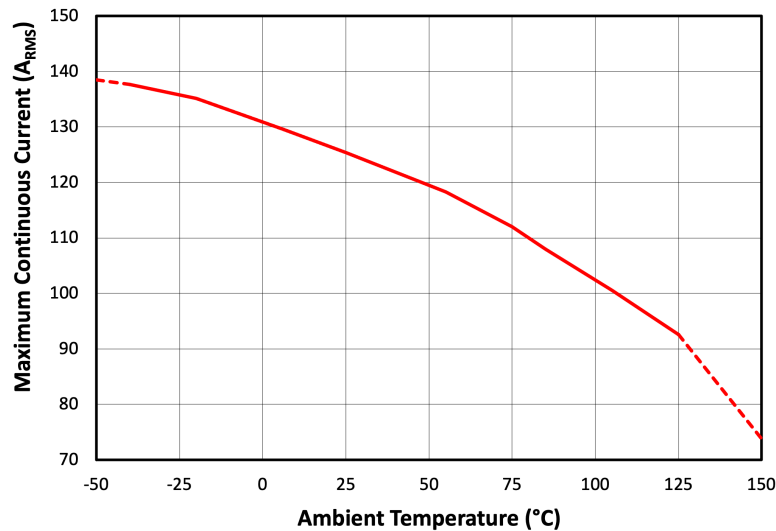
图 8-4. 最大连续 RMS 电流与环境温度间的关系
