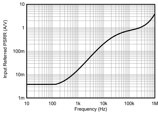
图 6-9. PSRR 与频率间的关系
