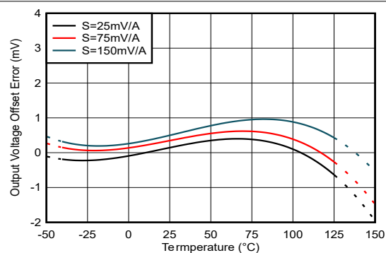
图 6-2. 失调误差与温度间的关系：TMCS1133Axx-Q1 器件选项
