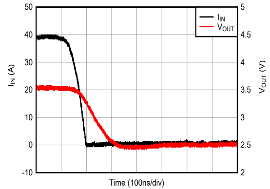
图 6-12. 电压输出阶跃响应 (下降)
