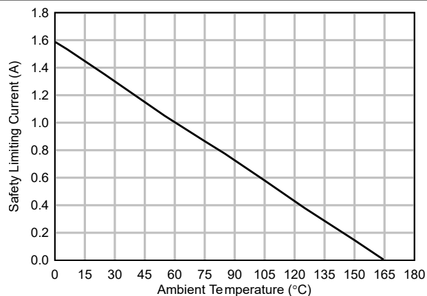
图 6-20. 安全限制电流的热降额曲线，侧 2
