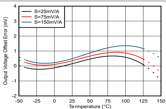
图 6-3. 失调误差与温度间的关系：TMCS1133Bxx-Q1 器件选项
