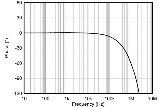
图 6-8. 相位与频率间的关系 (所有增益)
