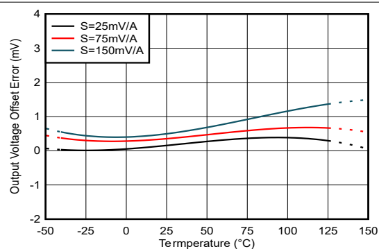
图 6-4. 失调误差与温度间的关系：TMCS1133Cxx-Q1 器件选项
