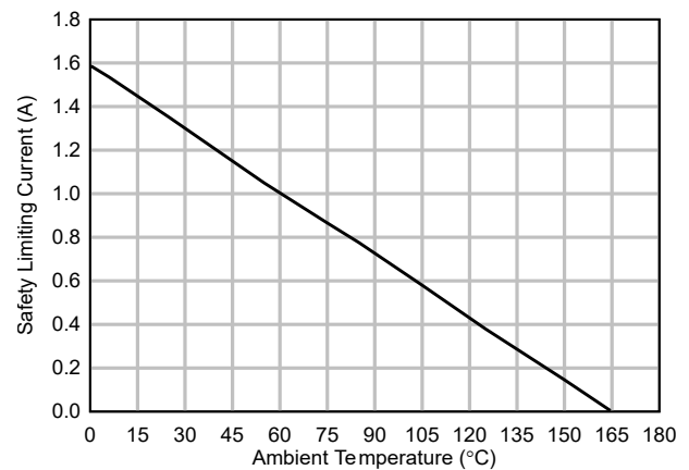
图 6-14. 安全限制电流的热降额曲线，侧 2
