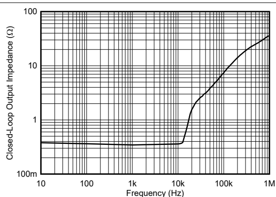
图 6-4. 输出阻抗与频率间的关系
