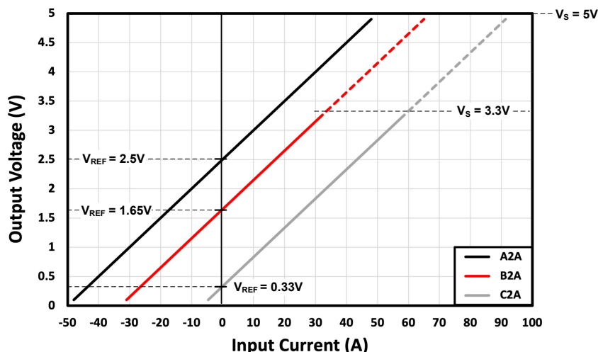
图 8-3. TMCS11xxx2A 的输出电压与输入电流之间的关系
