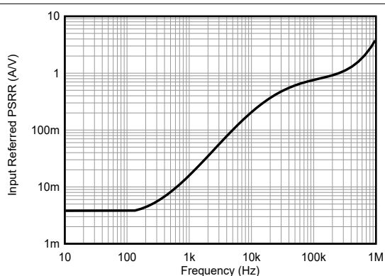
图 6-3. PSRR 与频率间的关系
