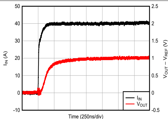
图 6-9. 电压输出阶跃响应 (上升)
