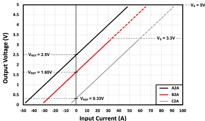
图 8-5. TMCS11xxx2A-Q1 的输出电压与输入电流之间的关系
