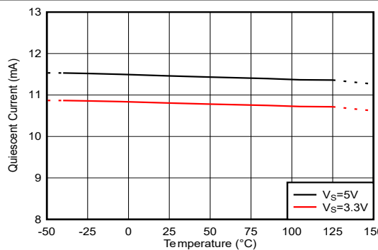
图 6-14. 静态电流与温度间的关系
