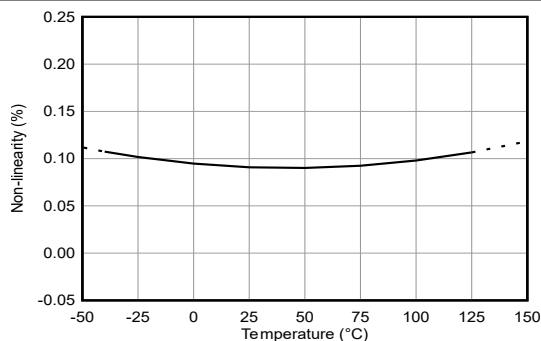
图 6-3. 非线性与温度间的关系
