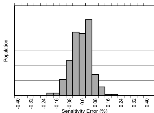
图 6-4. 灵敏度误差产生分布图：A 级
