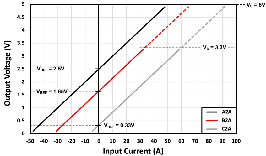
图 8-5. TMCS1126x2A 的输出电压与输入电流之间的关系
