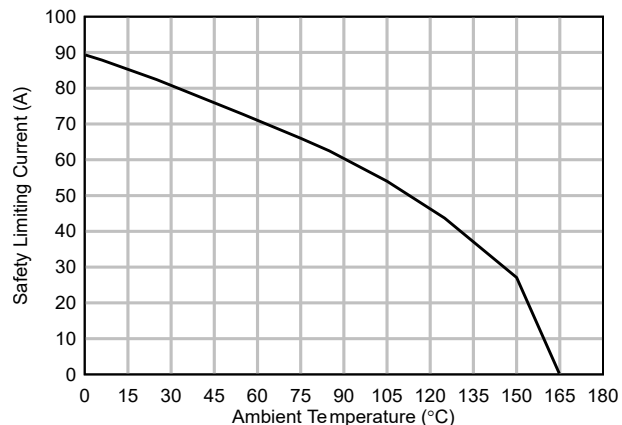
图 6-17. 安全限制电流的热降额曲线，侧 1
