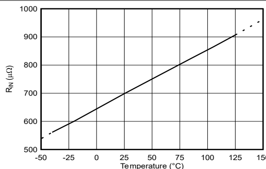
图 6-16. 输入导体电阻与温度间的关系
