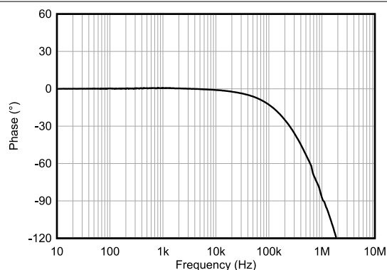
图 6-6. 相位与频率间的关系 (所有增益)
