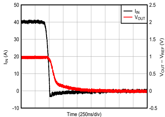
图 6-10. 电压输出阶跃响应 (下降)
