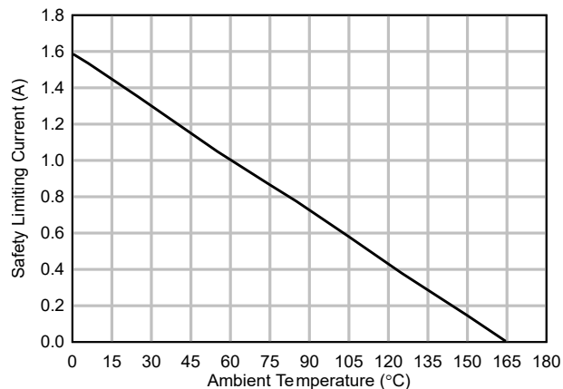
图 6-18. 安全限制电流的热降额曲线，侧 2
