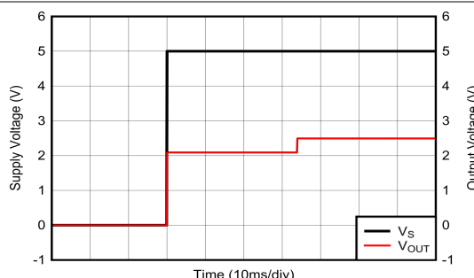
图 6-12. 启动瞬态响应
