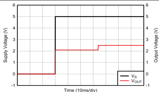
图 6-18. 启动瞬态响应
