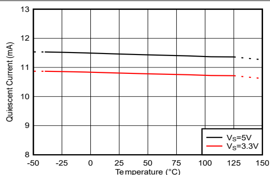
图 6-20. 静态电流与温度间的关系
