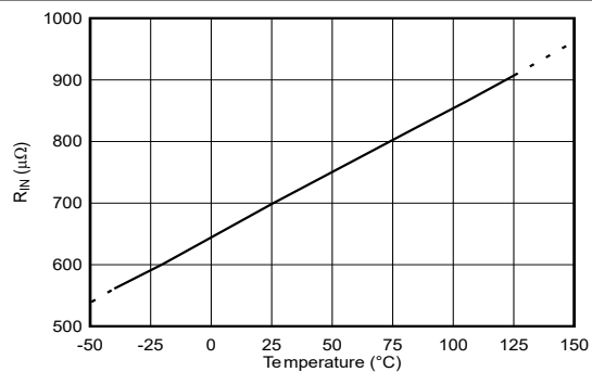
图 6-21. 输入导体电阻与温度间的关系
