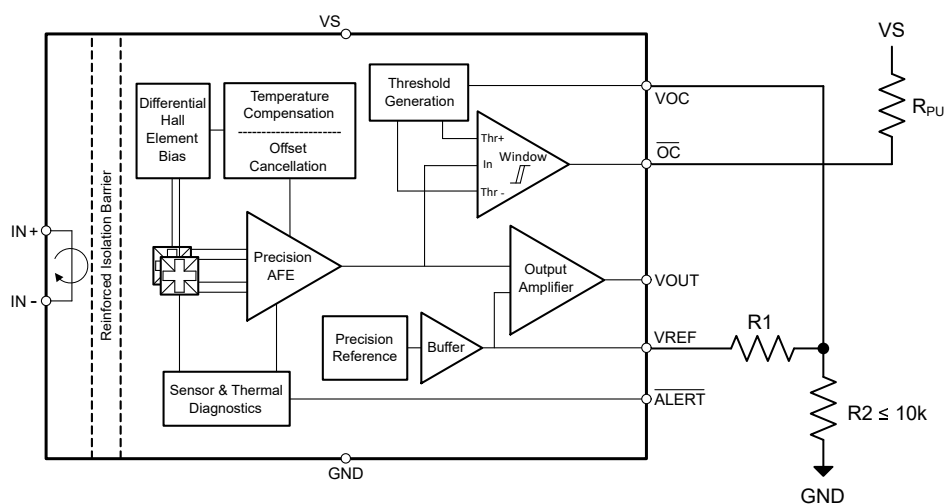
图 8-6. 使用零电流输出基准电压的用户可配置过流阈值
