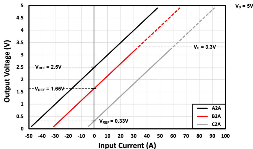
图 8-4. TMCS1123x2A-Q1 的输出电压与输入电流之间的关系
