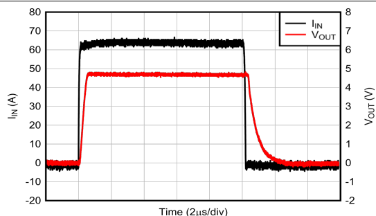
图 6-17. 电流过载响应
