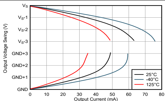
图 6-19. 输出摆幅与输出电流间的关系
