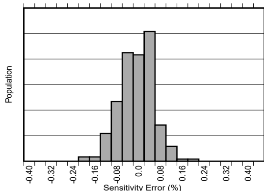
图 6-5. 灵敏度误差产生分布图
