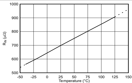
图 6-22. 输入导体电阻与温度间的关系
