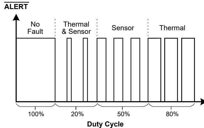
图 8-10. 传感器诊断波形
