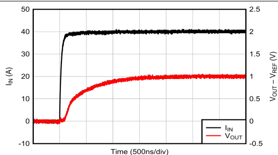
图 6-15. 电压输出阶跃响应 (上升)
