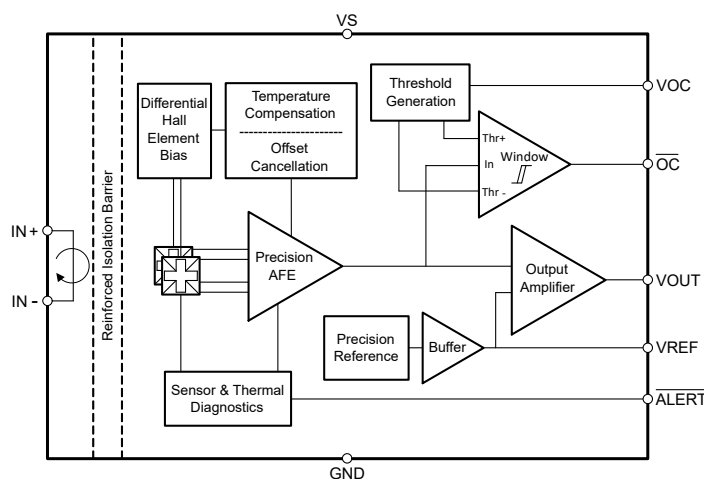
图 8-1. 功能方框图
