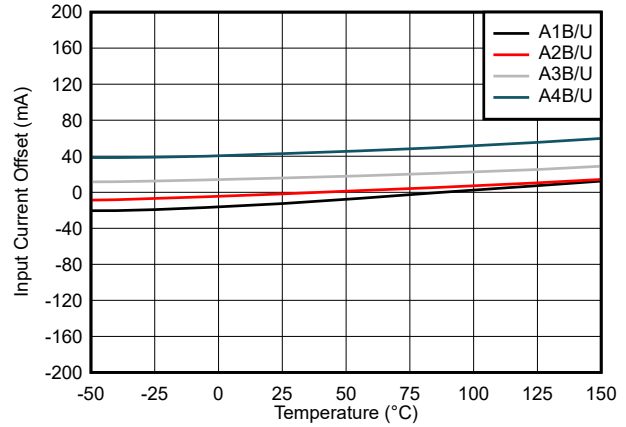
图 7-2. TMCS1107 输入失调电流与温度间的关系
