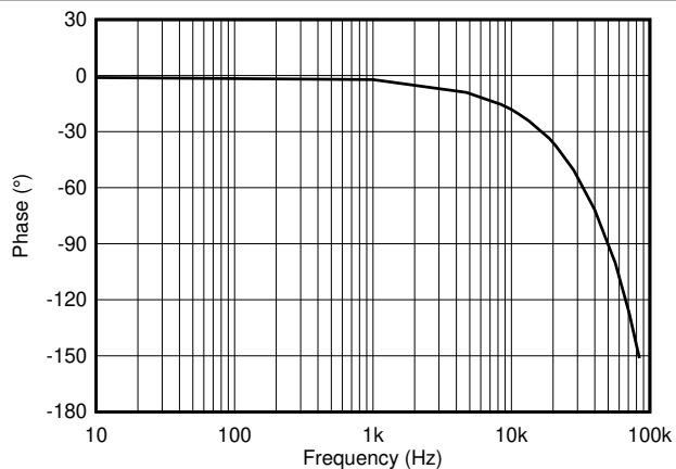
图 6-18. 相位与频率间的关系 (所有增益)
