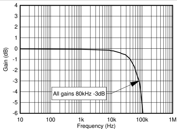
图 6-17. 灵敏度与频率间的关系 (所有增益都归一化为 1Hz)
