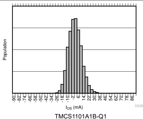
图 6-9. 输入偏移电流产生分布图
