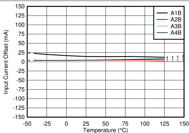
图 8-2. 整个温度范围内的失调误差漂移 (B 型号)
