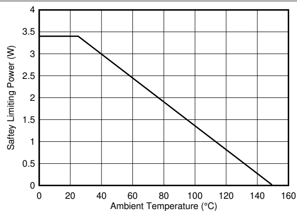
图 6-30. 安全限制功率的热降额曲线
