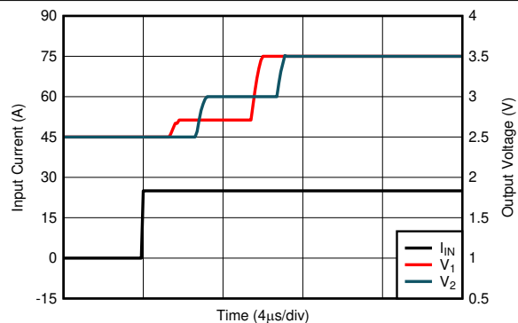
图 6-23. 电压输出阶跃 (上升)
