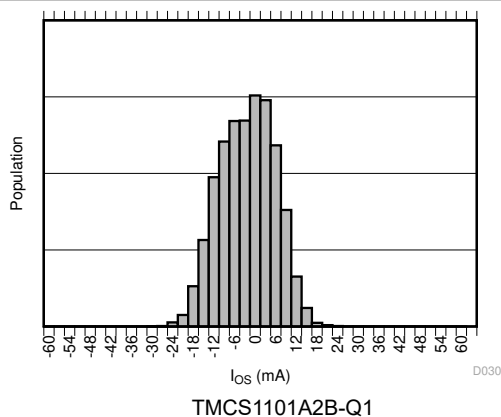
图 6-11. 输入偏移电流产生分布图
