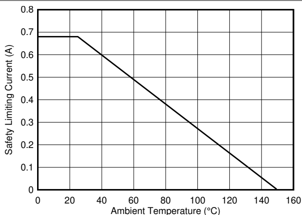
图 6-29. 安全限制电流的热降额曲线，侧 2
