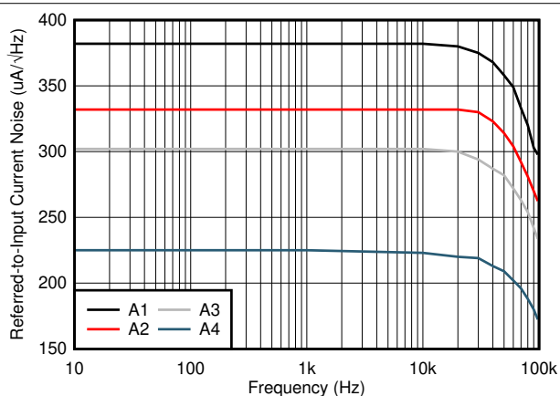
图 6-22. 以输入为基准的噪声与频率间的关系
