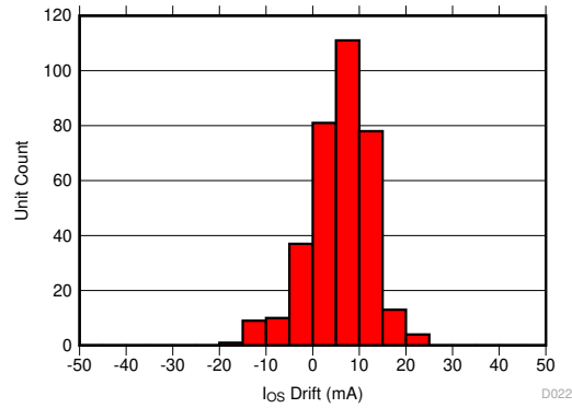
图 8-8. AEC-Q100 高温工作寿命应力测试后的以输入为基准的失调漂移
