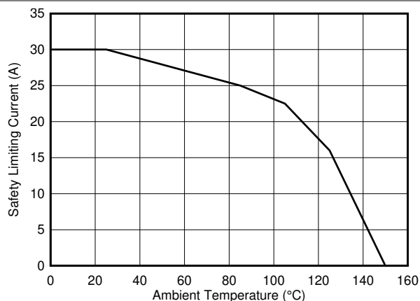
图 6-28. 安全限制电流的热降额曲线，侧 1
