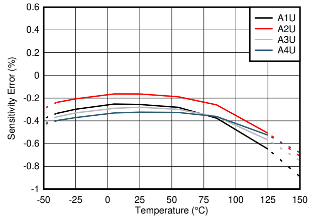
图 8-5. 整个温度范围内的灵敏度漂移 (U 型号)
