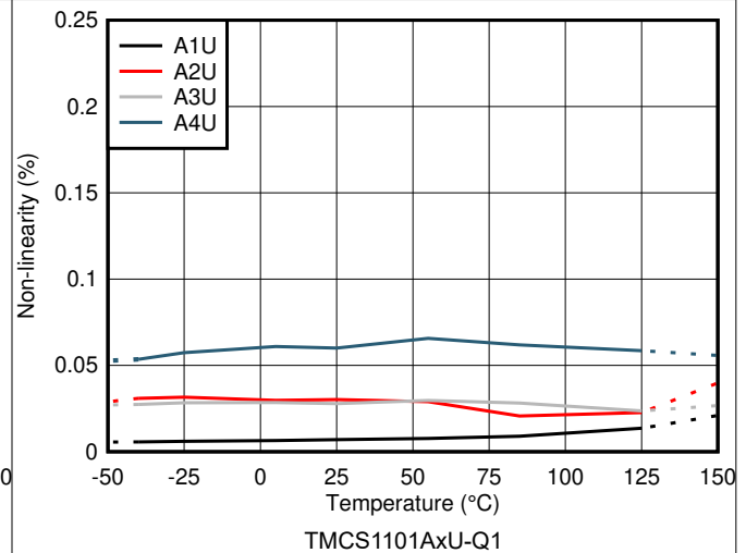
图 6-6. 非线性与温度间的关系
