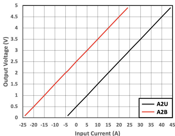
图 8-14. TMCS1101A2B-Q1 和 TMCS1101A2U-Q1 输出电压与输入电流的关系
