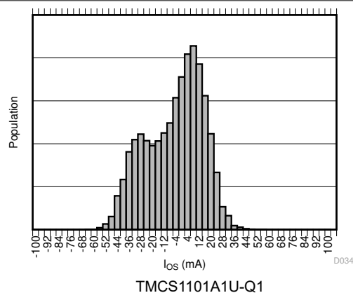
图 6-10. 输入偏移电流产生分布图
