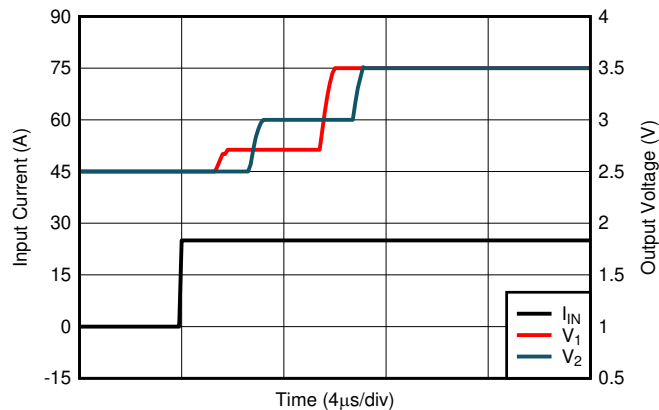
图 8-12. 对足以产生 1V 输出摆幅的输入电流阶跃的瞬态响应
