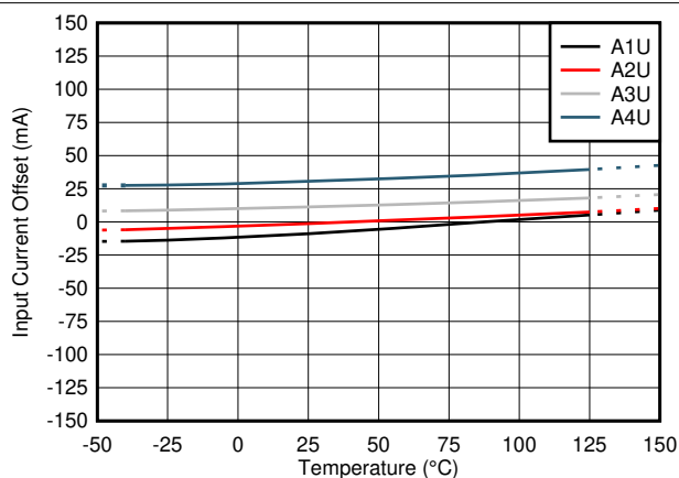
图 8-3. 整个温度范围内的失调误差漂移 (U 型号)
