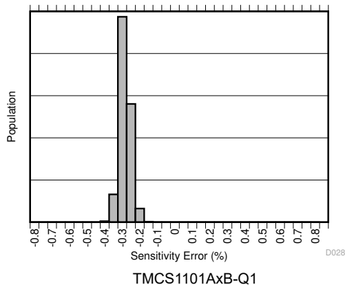
图 6-7. 灵敏度误差产生分布图
