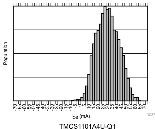
图 6-16. 输入偏移电流产生分布图
