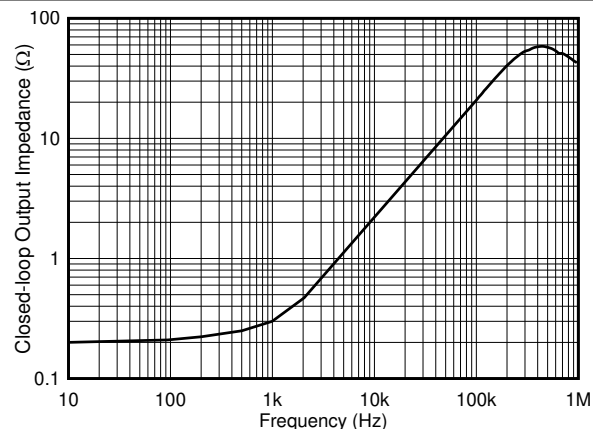
图 6-20. 输出阻抗与频率间的关系
