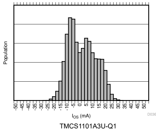
图 6-14. 输入偏移电流产生分布图
