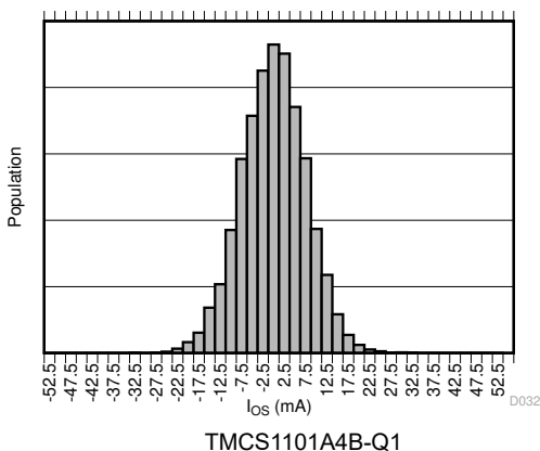
图 6-15. 输入偏移电流产生分布图
