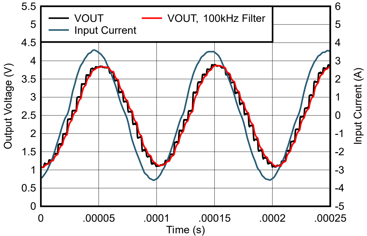
图 8-11. 对 10kHz 正弦波输入电流的响应行为
