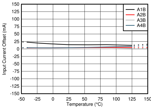
图 6-3. TMCS1101AxB-Q1 输入失调电流与温度间的关系
