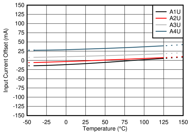
图 6-4. TMCS1101AxU-Q1 输入失调电流与温度间的关系
