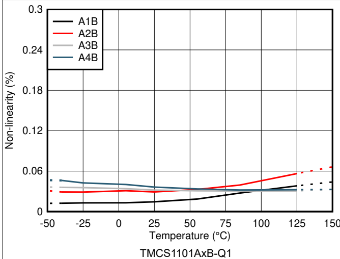
图 6-5. 非线性与温度间的关系
