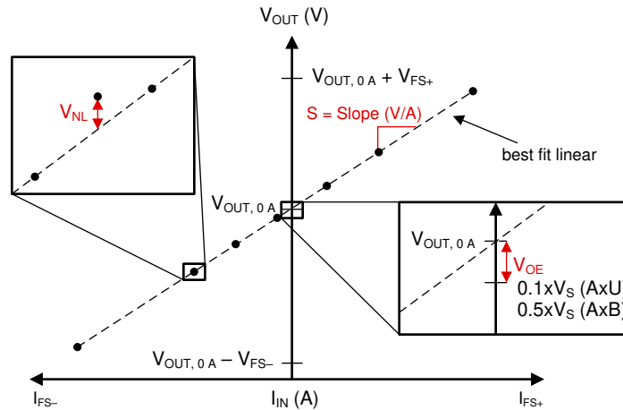
图 7-1. 灵敏度、失调电压和非线性误差
