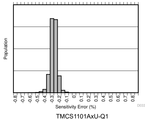
图 6-8. 灵敏度误差产生分布图
