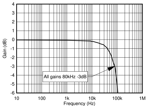
图 8-9. 归一化增益，所有型号
