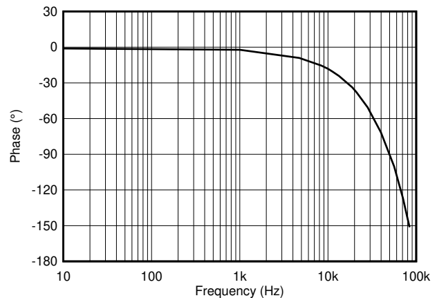
图 8-10. 归一化相位，所有型号
