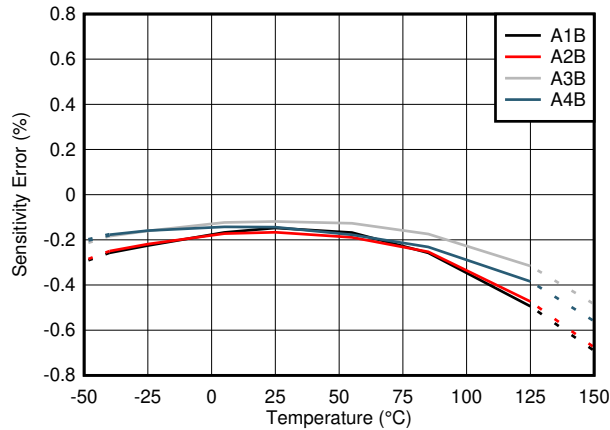
图 6-1. TMCS1101AxB-Q1 灵敏度误差与温度间的关系
