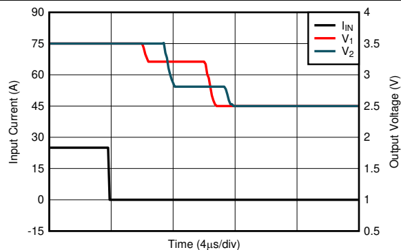
图 6-24. 电压输出阶跃 (下降)
