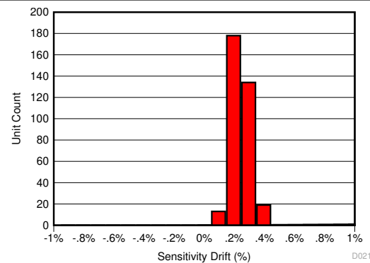
图 8-7. AEC-Q100 高温工作寿命应力测试后的灵敏度误差漂移
