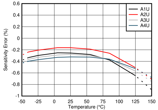
图 6-2. TMCS1101AxU-Q1 灵敏度误差与温度间的关系
