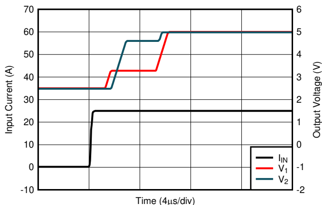
图 8-13. 对大输入电流阶跃的瞬态响应
