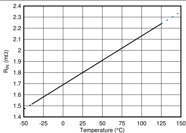
图 6-27. 输入导体电阻与温度间的关系
