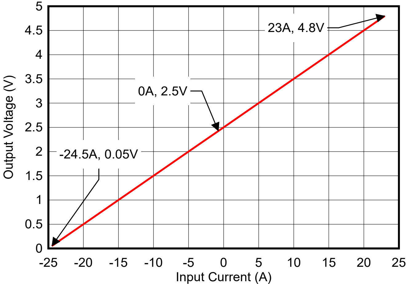
图 9-3. 应用示例设计传递曲线
