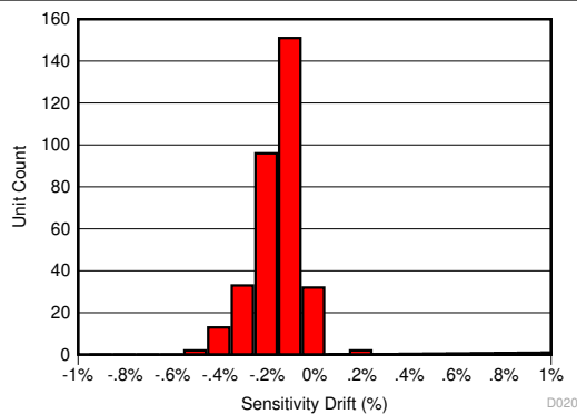
图 8-6. 130°C、85% RH HAST 后的灵敏度误差
