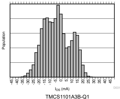
图 6-13. 输入偏移电流产生分布图
