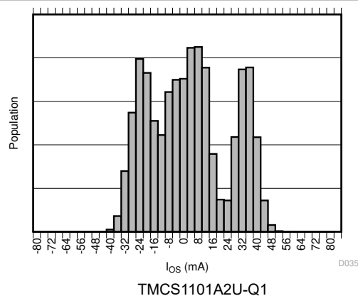
图 6-12. 输入偏移电流产生分布图
