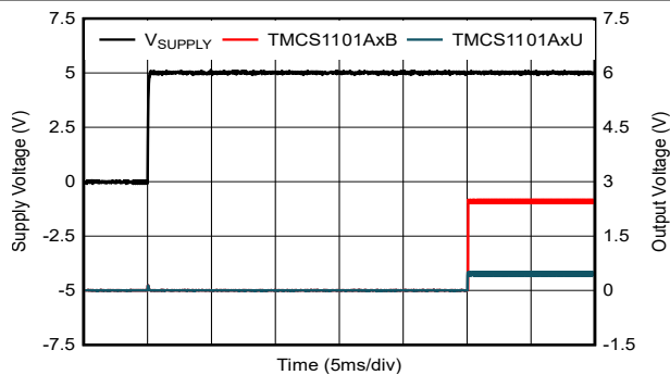
图 6-26. 启动瞬态响应
