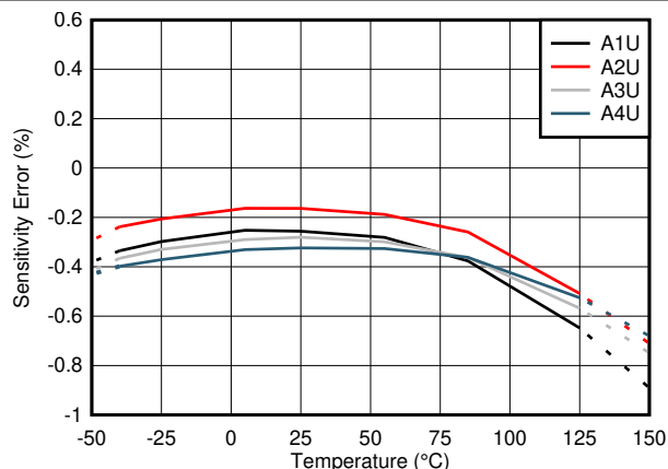
图 9-5. 整个温度范围内的灵敏度漂移 (U 型号)
