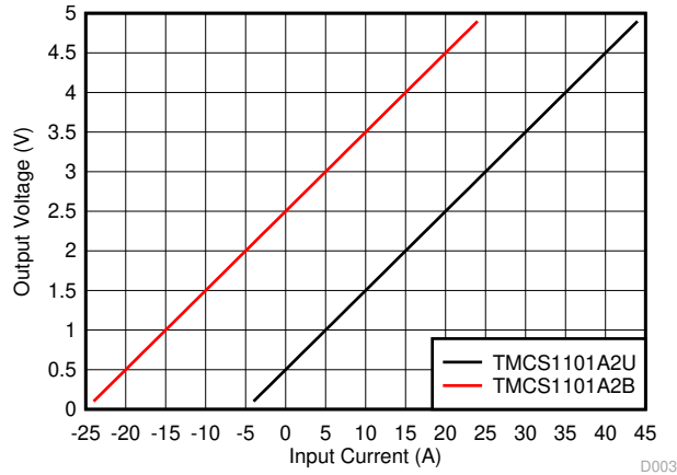
图 9-14. TMCS1101A2B 和 TMCS1101A2U
