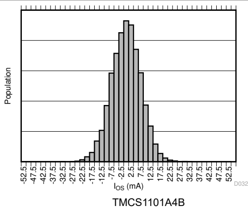
图 7-15. 输入失调电流产生分布
