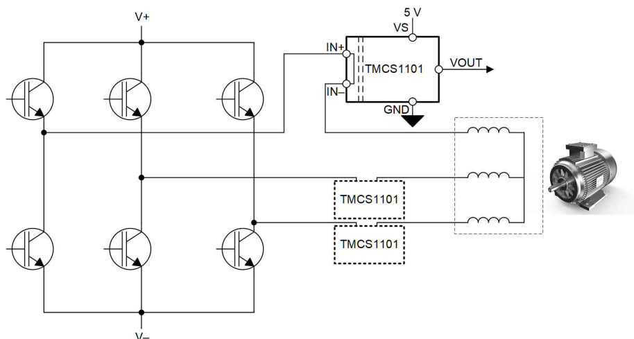
图 10-2. 内联电机相电流感测
