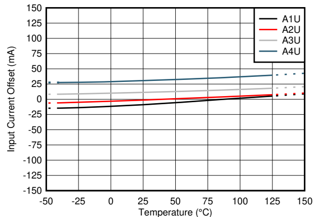
图 9-3. 整个温度范围内的失调误差漂移 (U 型号)
