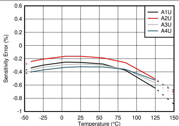
图 7-2. TMCS1101AxU 灵敏度误差与温度间的关系
