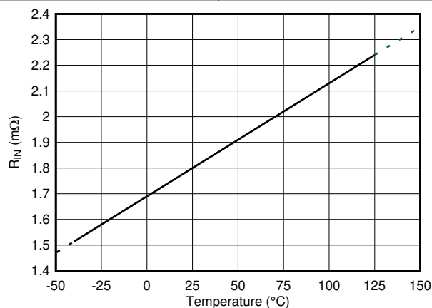
图 7-27. 输入导体电阻与温度间的关系
