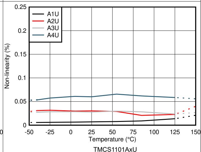
图 7-6. 非线性与温度间的关系
