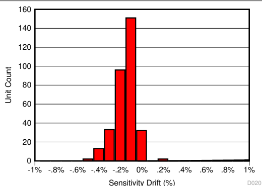
图 9-6. 130°C、85% RH HAST 后的灵敏度误差
