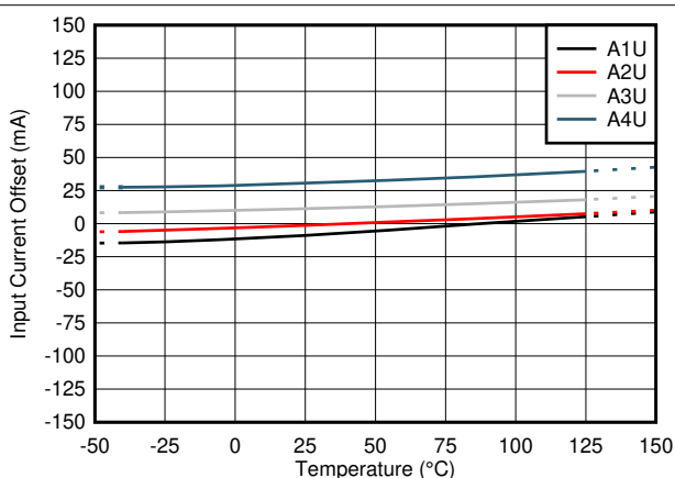
图 7-4. TMCS1101AxU 输入失调电流与温度间的关系
