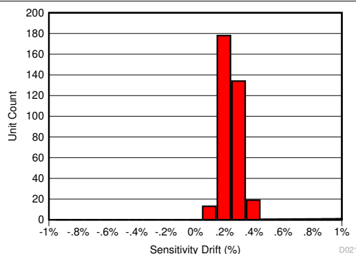
图 9-7. AEC-Q100 高温工作寿命应力测试后的灵敏度误差漂移
