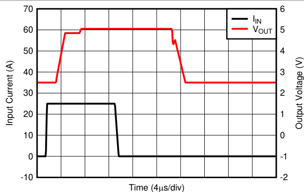
图 7-25. 电流过载响应
