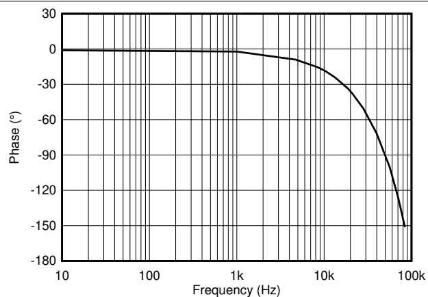
图 7-18. 相位与频率间的关系 (所有增益)
