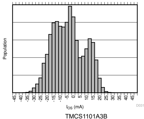
图 7-13. 输入失调电流产生分布
