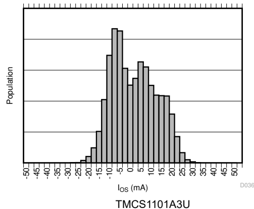
图 7-14. 输入失调电流产生分布
