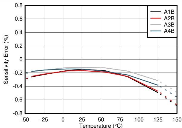
图 9-4. 整个温度范围内的灵敏度漂移 (B 型号)
