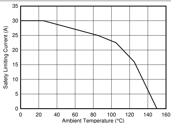
图 7-28. 安全限制电流的热降额曲线，侧 1
