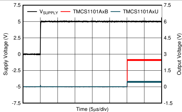
图 7-26. 启动瞬态响应
