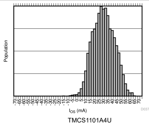
图 7-16. 输入失调电流产生分布
