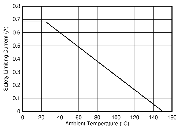
图 7-29. 安全限制电流的热降额曲线，侧 2
