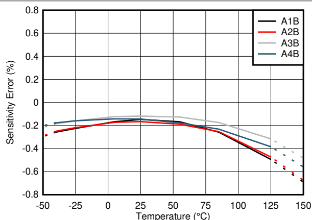
图 7-1. TMCS1101AxB 灵敏度误差与温度间的关系
