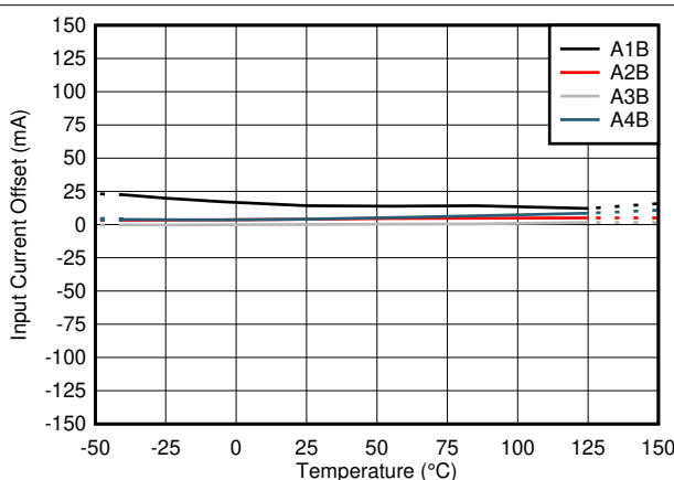
图 7-3. TMCS1101AxB 输入失调电流与温度间的关系
