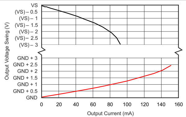
图 6-12. 输出摆幅与输出电流间的关系
