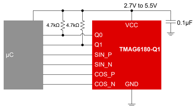
应用方框图
