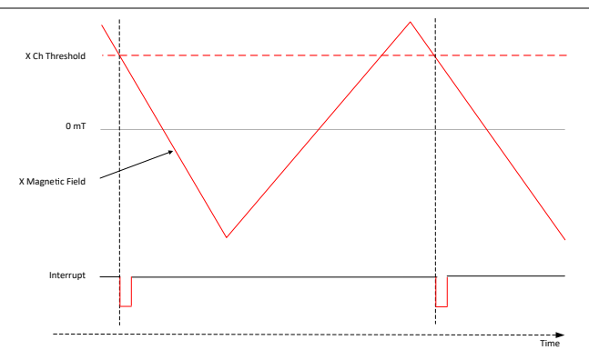
图 7-5. MAG_THR_DIR = 1b 番茄 THR_HYST = 000b 时的磁体下限交叉检查
