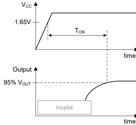
图 7-4. V_{CC} 斜坡的 T_{ON}
