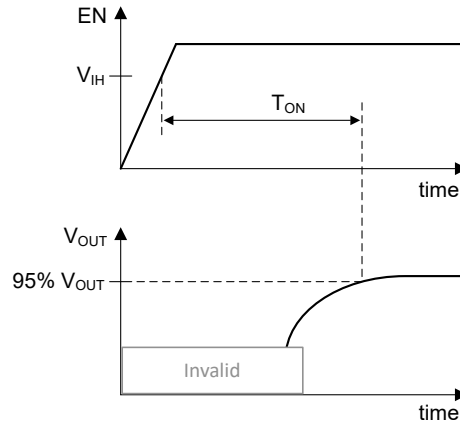
图 7-5. 使用 EN 引脚时的 T_{ON}
