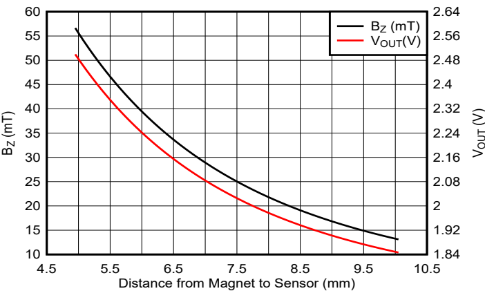
图 9-9. 磁场 (B Z ) 及传感器输出电压 (V OUT ) 与磁体到传感器的距离之间的关系
