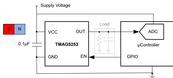
典型原理图
