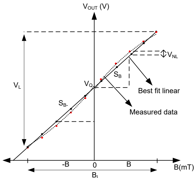
图 7-1. 磁响应的线性度 ( 双极 )
