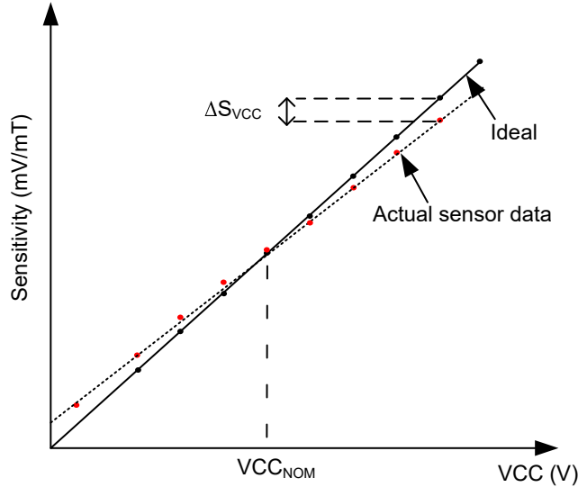
图 7-2. 灵敏度比例式误差
