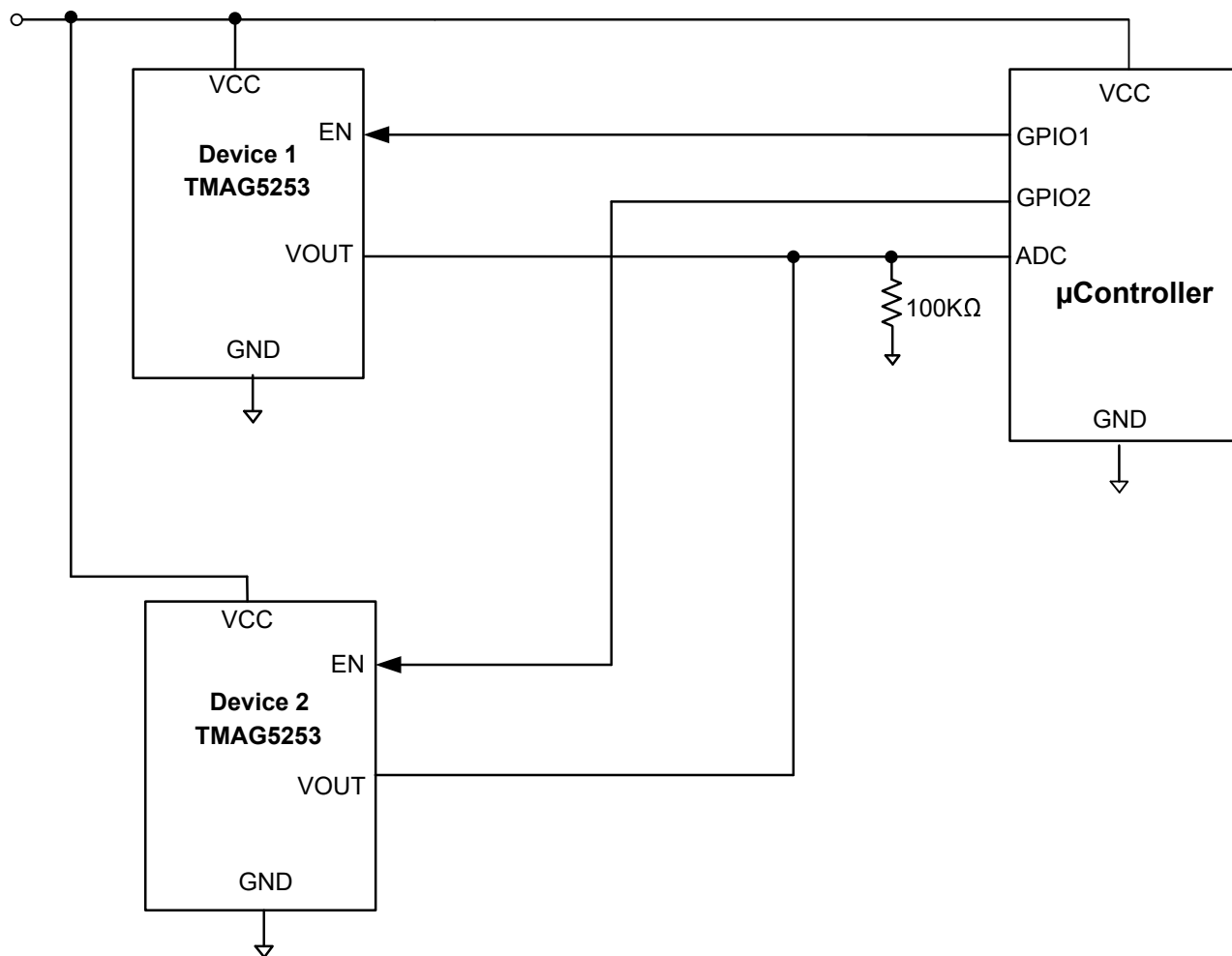
图 9-1. 多个使用共享输出的传感器
