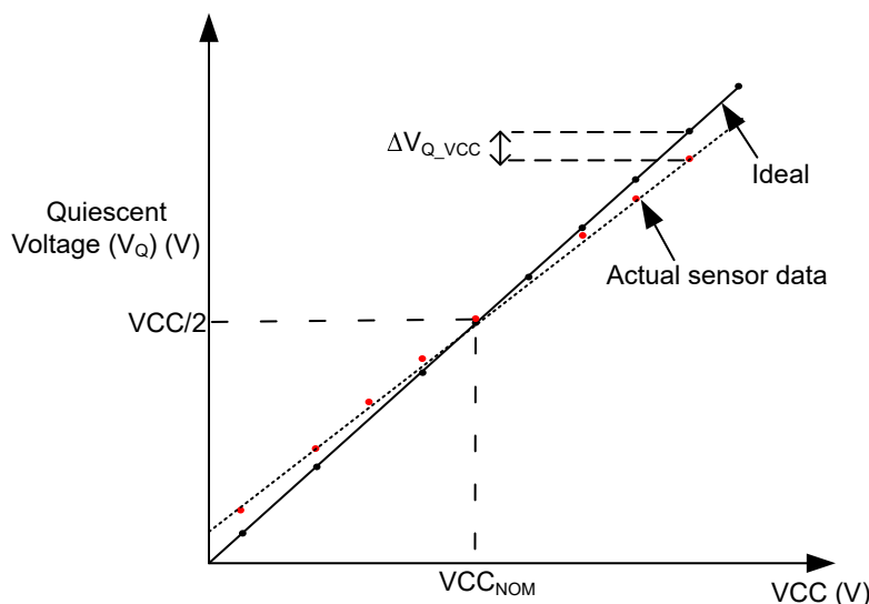
图 7-3. 静态电压比例式误差
