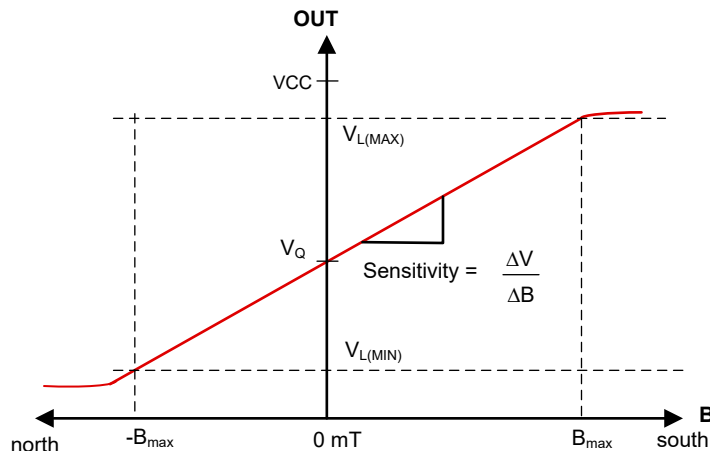
图 8-4. TMAG5253B ( 双极 ) 版本的磁响应
