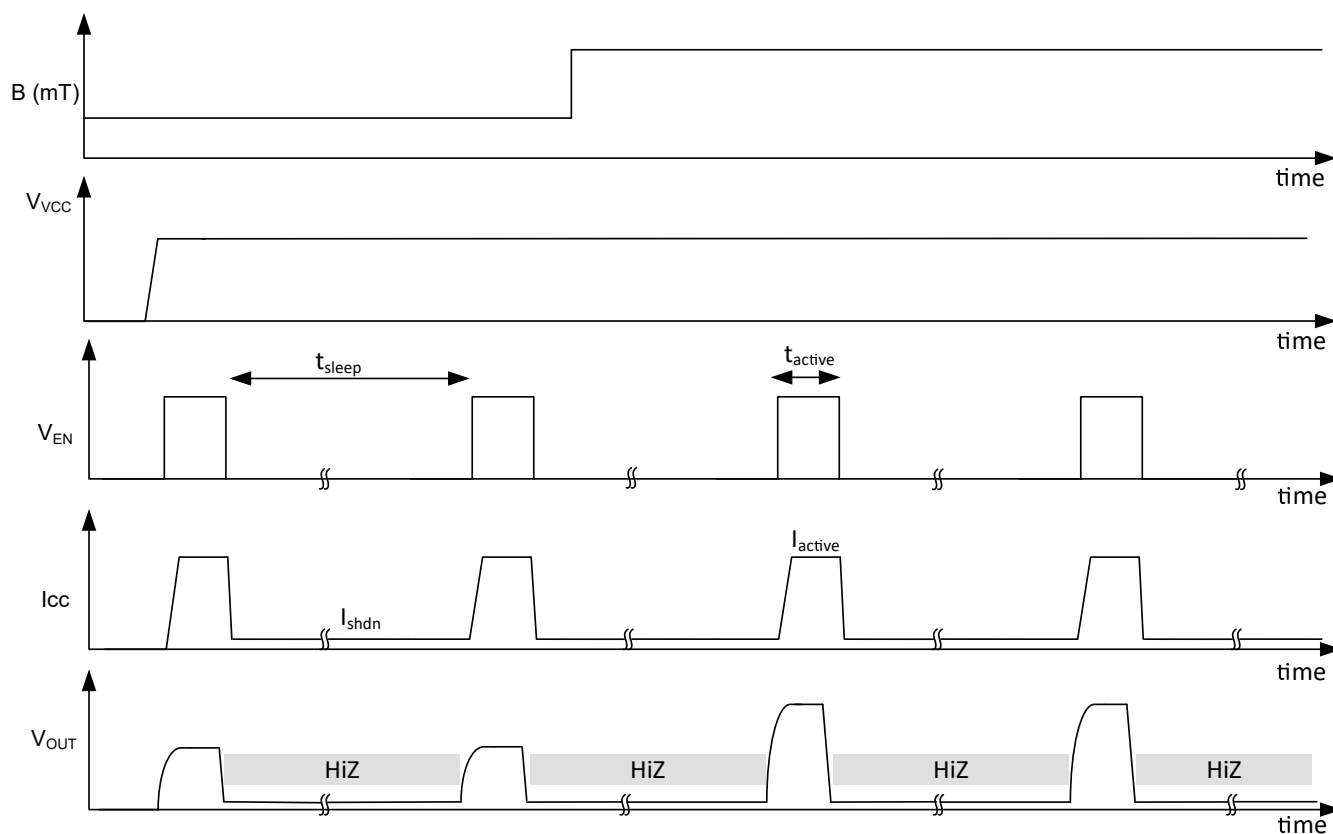
图 9-4. 占空比控制应用的时序图
