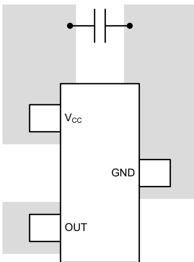
图 9-14. SOT-23 布局示例
