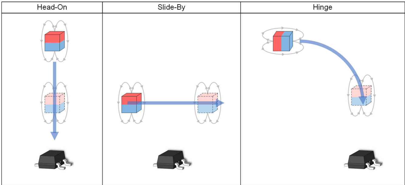
图 9-1. 设计实现方案
