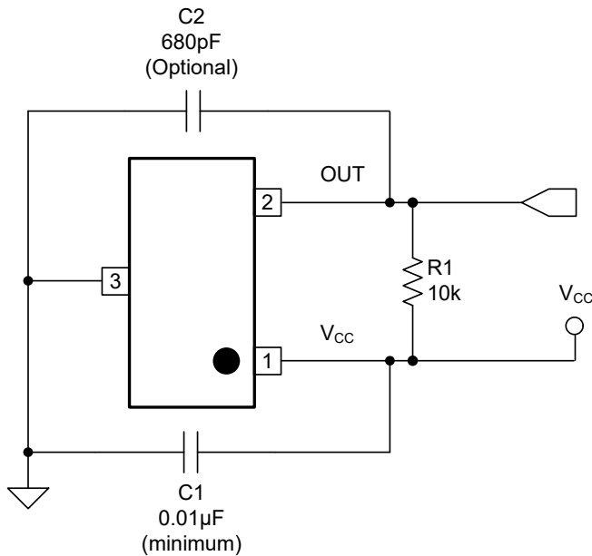
图 8-1. 典型应用电路
