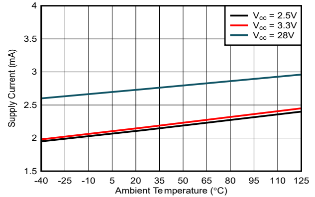
图 6-2. 30kHz：平均 I_{CC} 与温度间的关系
