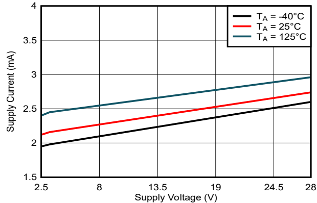
图 6-1. 30kHz：平均 I_{CC} 与 V_{CC} 间的关系
