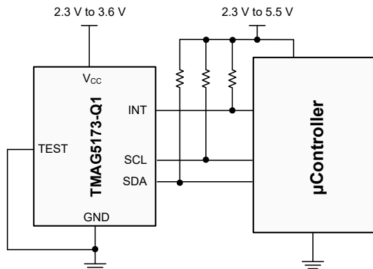
应用方框图
