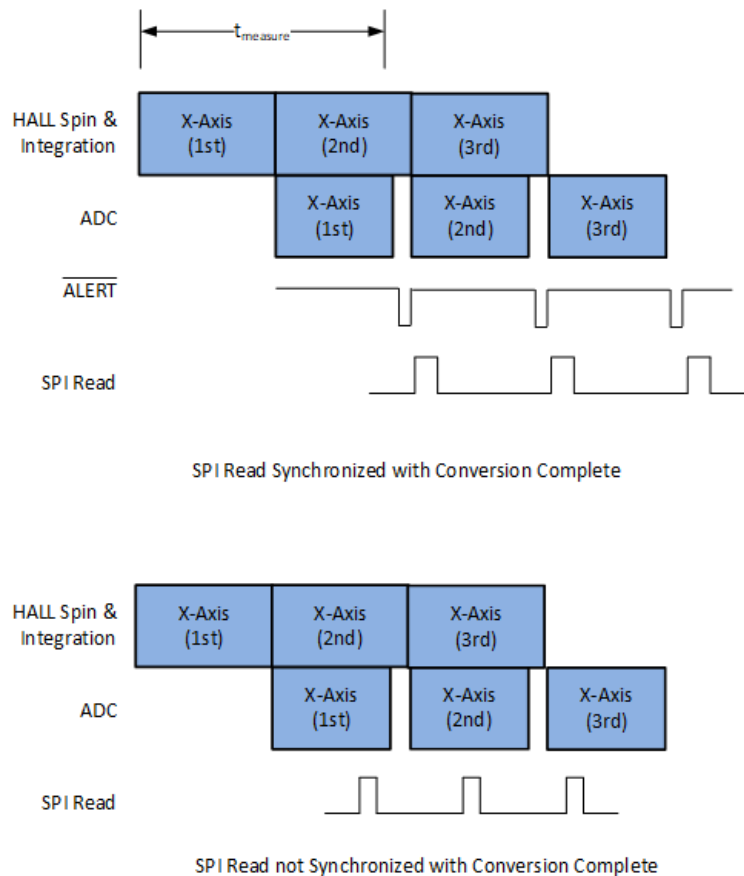
图 8-8. 连续转换期间的 SPI 读取
