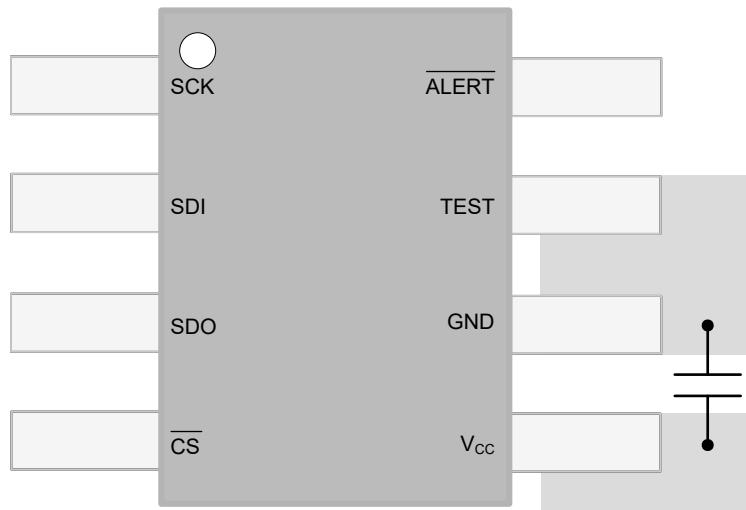
图 10-1. 布局示例 - TMAG5170-Q1
