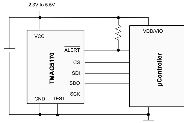
图 8-4. TMAG5170-Q1 应用示意图
