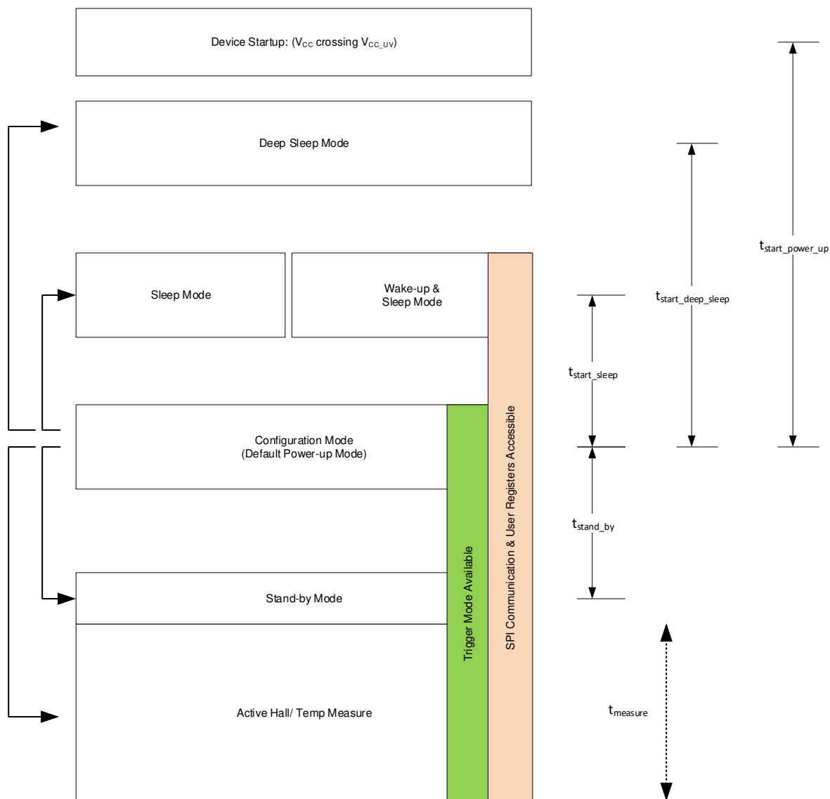
图 7-4. TMAG5170-Q1 上电序列
