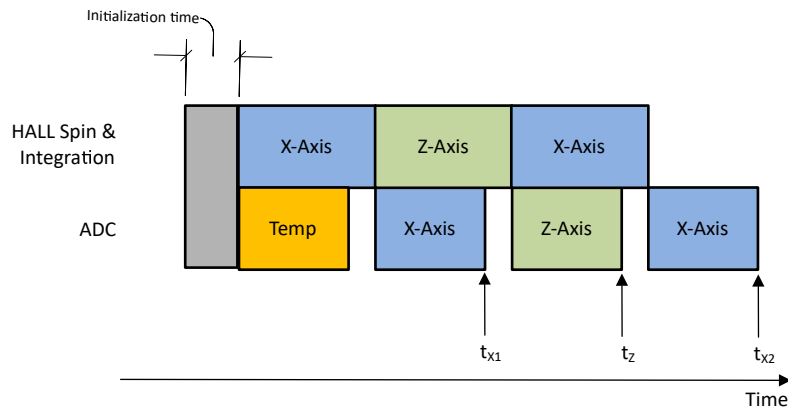
图 8-3. XZX 磁场转换
