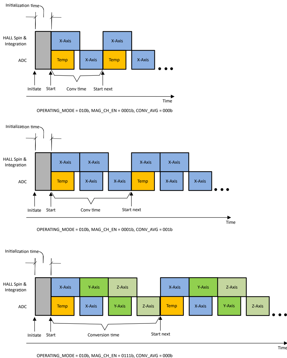
图 8-1. 连续转换模式
