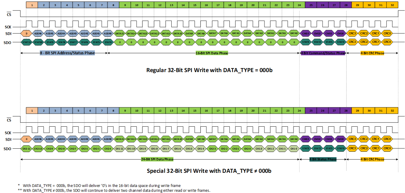
图 7-15. 32 位写入帧
