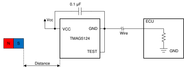
典型电路原理图
