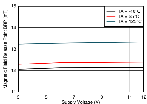
图 7-22. B_{RP} vs V_{CC}
