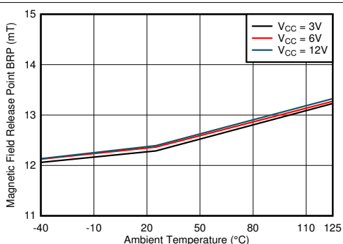
图 7-21. B_{RP} vs Temperature
