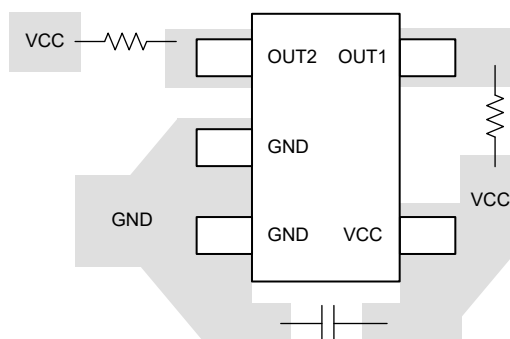
图 8-5. 布局示例 ( 引脚排列版本 : R )
