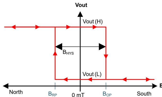
图 7-2. 锁存器功能
