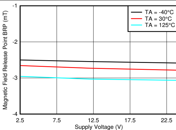
图 7-53. B_{RP\_Y} 阈值与 V_{CC}
