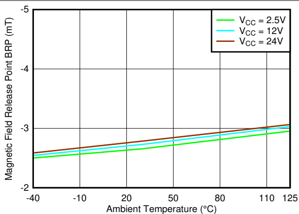
图 7-54. B_{RP\_Y} 阈值与温度
