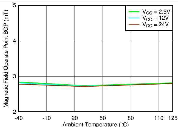
图 7-52. B_{OP\_Y} 阈值与温度
