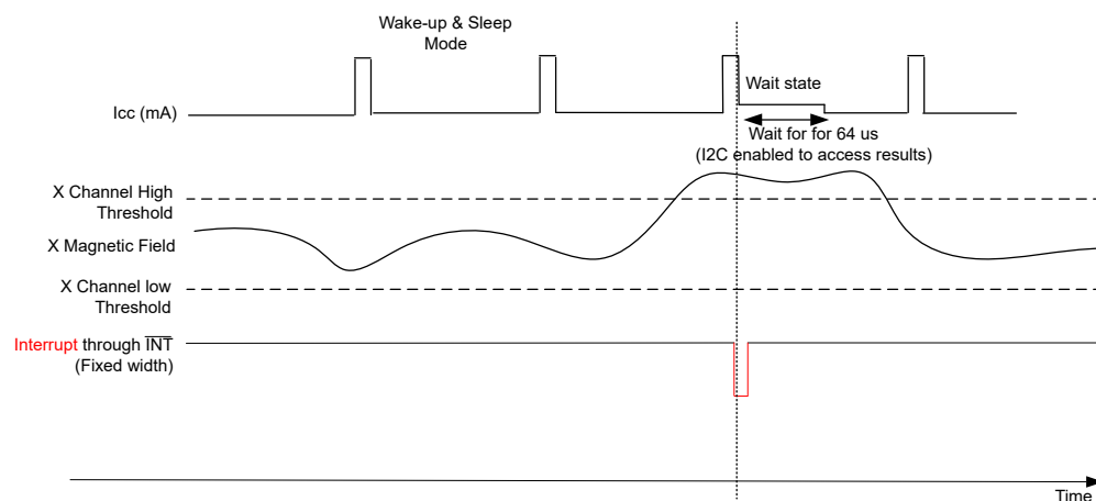
图 6-4. 通过 \overline{\text{INT}} 实现固定宽度中断
