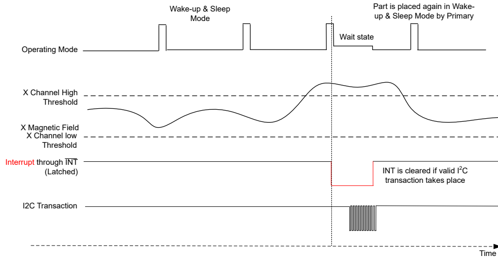
图 6-5. 通过 \overline{\text{INT}} 实现锁存中断
