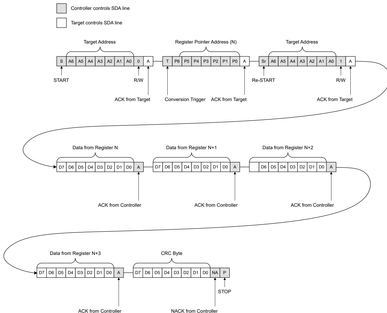
图 6-17. 标准 I 2 C 读取 (启用 CRC)
