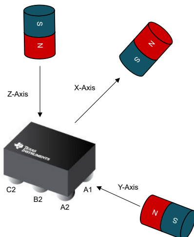
图 6-1. 灵敏度方向
