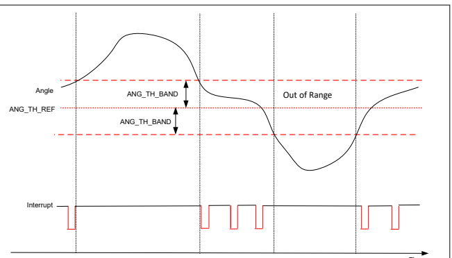
图 8-9. MAG_THR_DIR = 1b 、 THR_SEL=01b 、 INT_STATE=1b 时的角度限值交叉检查
