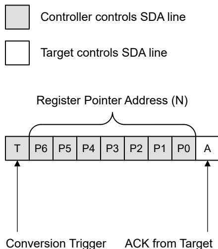
图 6-13. 控制寄存器
