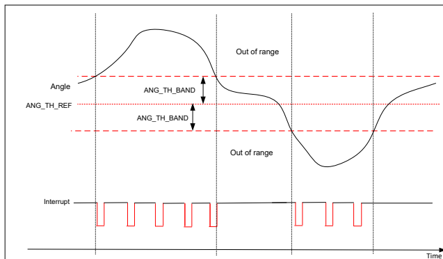
图 8-8. MAG_THR_DIR = 0h 、 THR_SEL[1:0] = 1h 、 INT_STATE = 1h 时的角度限值检查
