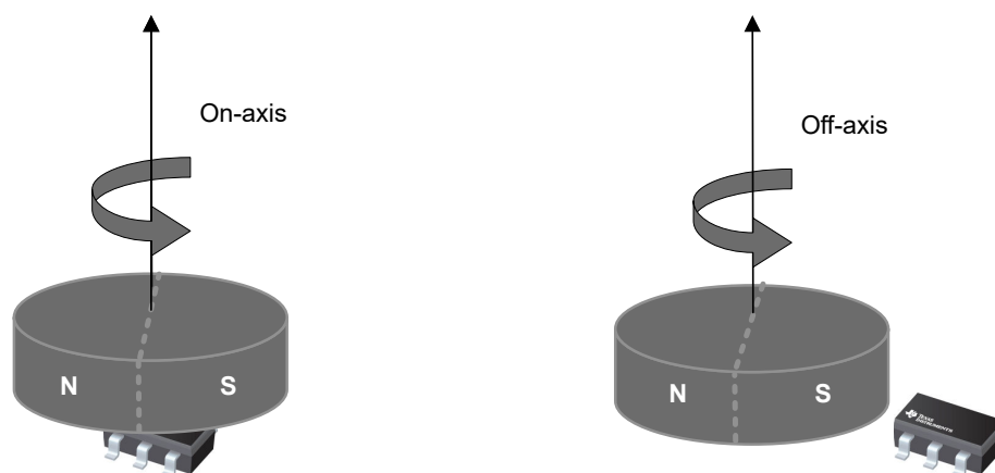
图 8-19. 同轴角度测量与离轴角度测量
