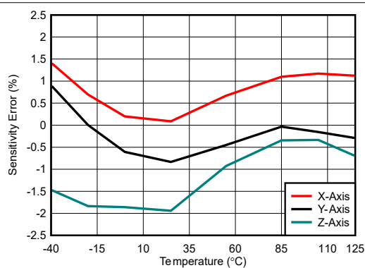
图 5-5. A2 灵敏度误差与温度间的关系, V_{CC} = 1.8V
