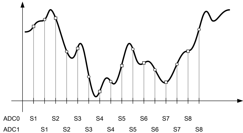
图 13-5. 交错采样
