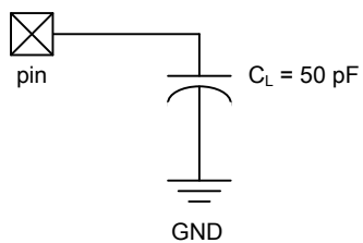
图 23-1. Load Conditions
