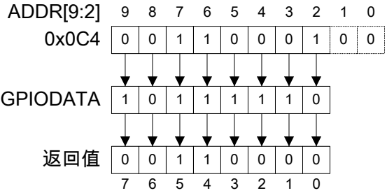
图 10-4. GPIODATA 读实例
