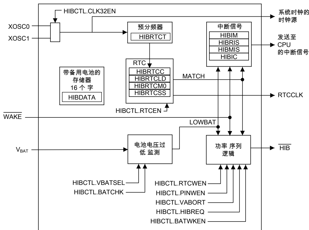
图 7-1. 休眠模块结构图
