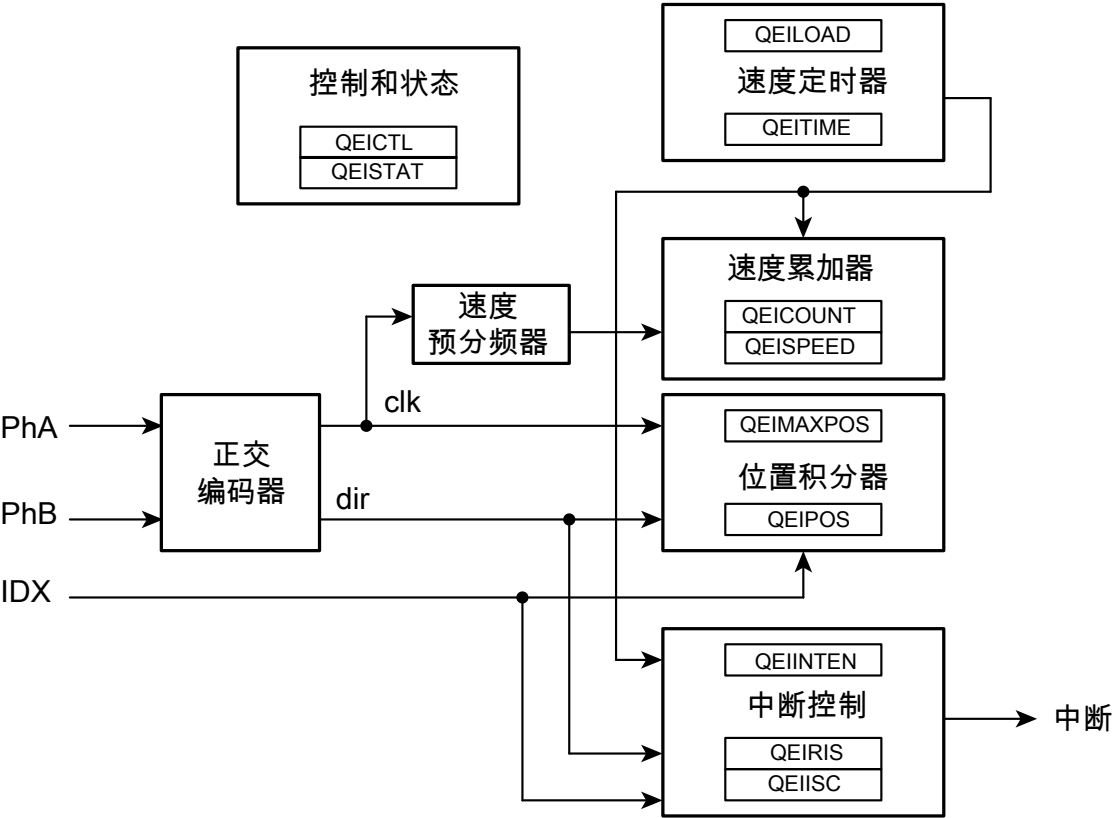
图 21-1. QEI结构图
