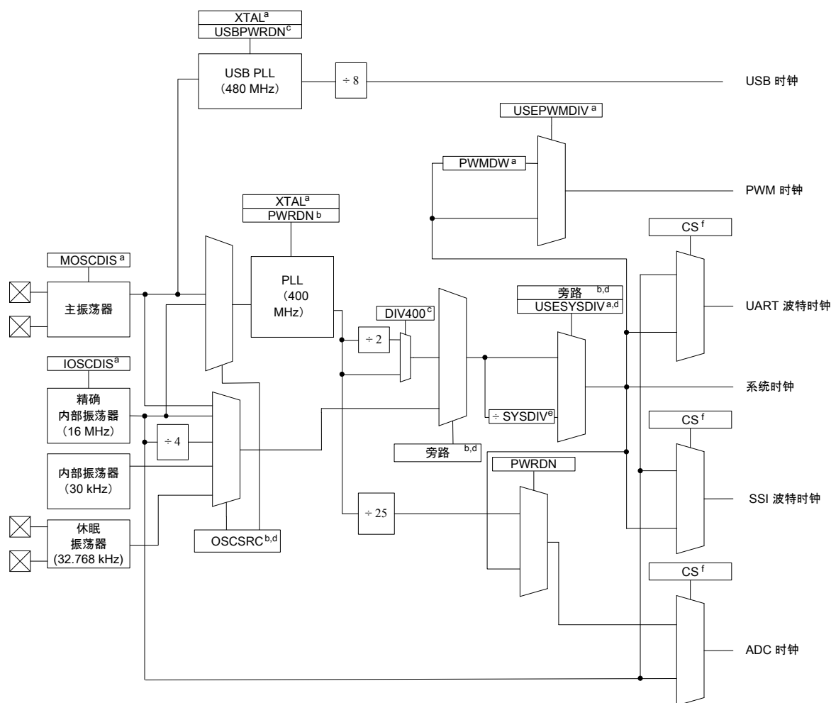
图 5-5. 主时钟树
