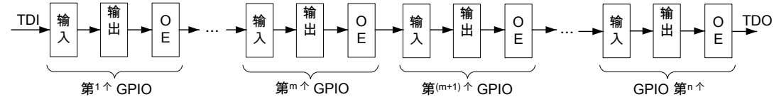
图 4-5. 边界扫描寄存器格式
