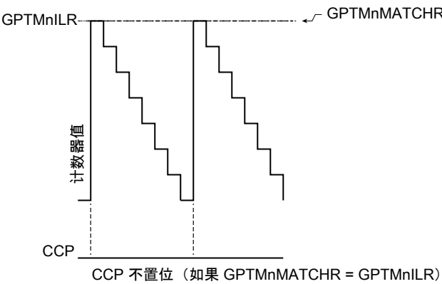
图 11-7. CCP 输出，GPTMTnMATCHR = GPTMTnILR
