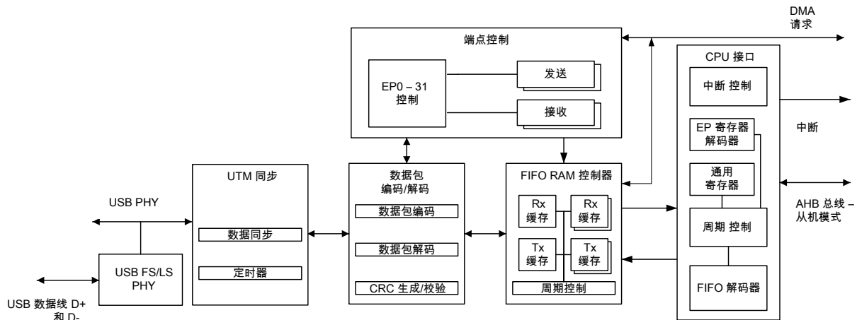
图 17-1. USB 模块结构图
