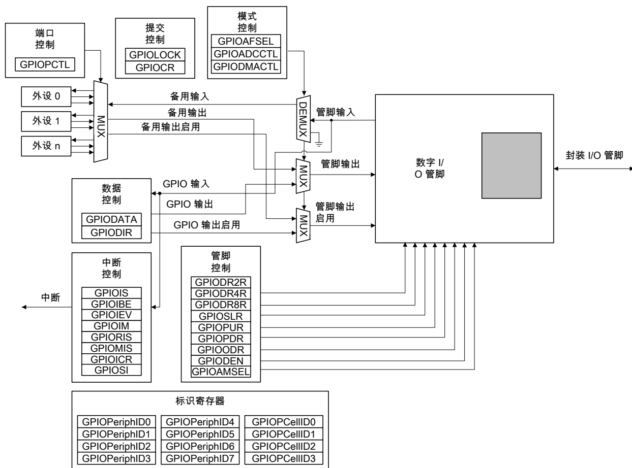
图 9-1. 数字 I/O 口
