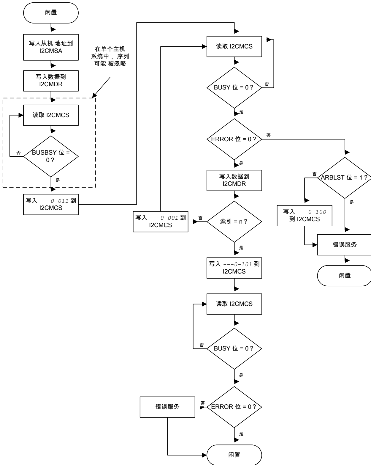
图 15-10. 多数数据字节的主机传输
