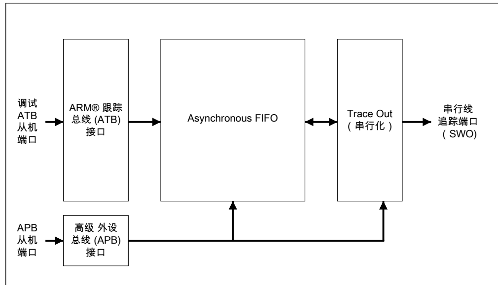
图 2-2. TPIU 方框图
