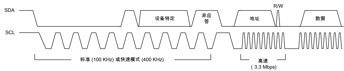
图 16-7. 高速数据格式
