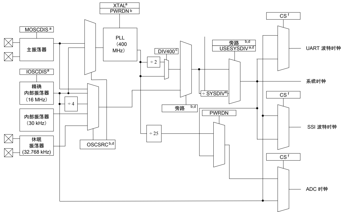
图 5-5. 主时钟树
