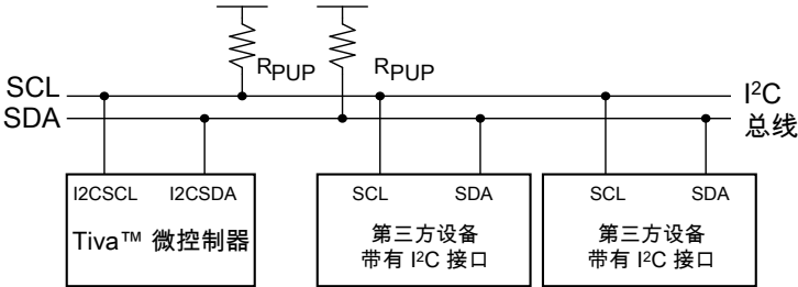
图 16-2. I 2 C 总线配置
