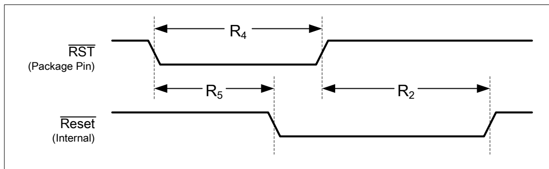
图 21-11. External Reset Timing ( \overline{\text{RST}} )
