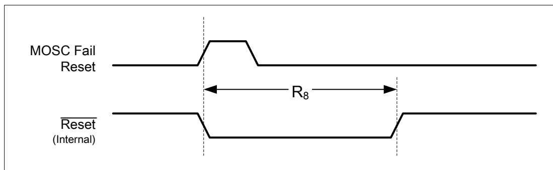
图 21-14. MOSC Failure Reset Timing
